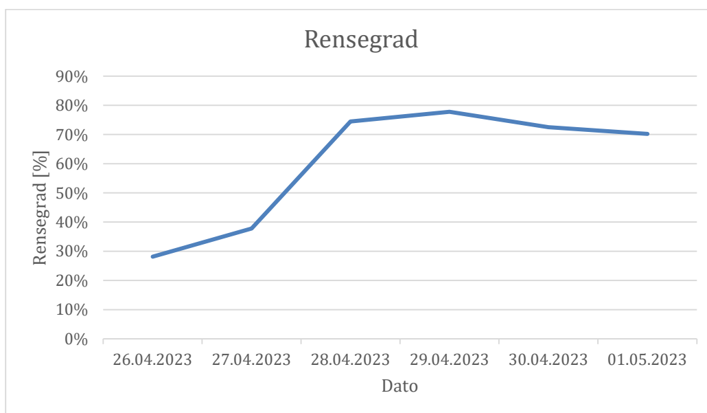
Figure 29. Beregnet rensgrad av nitrat i F1 via data fra loggere i feltet under metanolforsøket i uke 17 2023.
