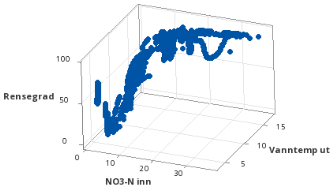
Figur 37. Plot som illustrerer sammenhengen mellom nitrat i forkammeret og vanntemperaturen ut av filteret i perioden april-september 2022. Høyeste konsentrasjonene av nitrat fra forkammeret kommer inn i biofilteret med høyere temperaturer (gunstig for anaerob denitrifikasjon). Dette medfører at det tilsynelatende ser ut til at rensegraden for nitrat i biofilteret er mest optimal ved høye input av nitrat til filteret, noe som sannsynligvis ikke stemmer. Data er fra loggere.
