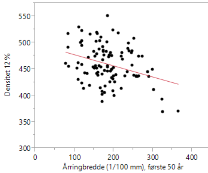
Figur 16 Densitet ( \text{kg/m}^3 ) forklart ved trees gjennomsnittlige årringbredde, for middels bonitet.
