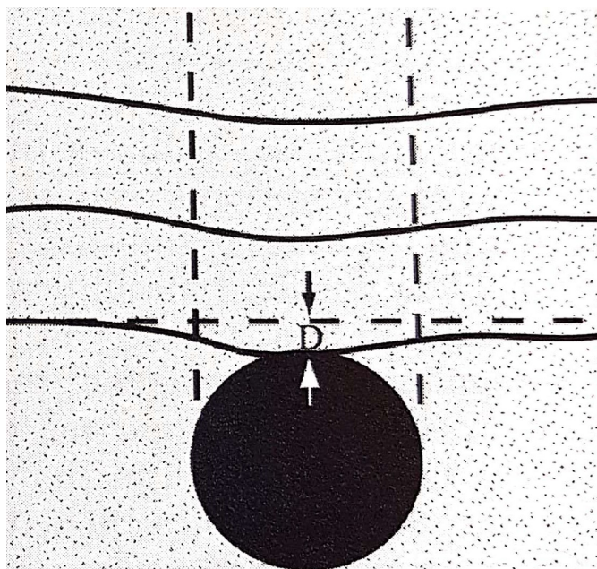
Figur 1.5: Korleis jordlasta påverkar fleksible røyr, og korleis setningane i jorda blir. D representerar deformasjonen til det fleksible røyrret. (Moser, 2001)
