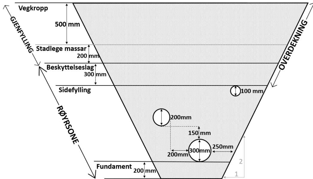
Figur 2.4: Utgangspunkt for analysa til fleirrørsgrofter. Rørstorleik og mål i rørsona er likt for alle variablar av grøfta, med unntak av grøftehelling og gjenfylling.
