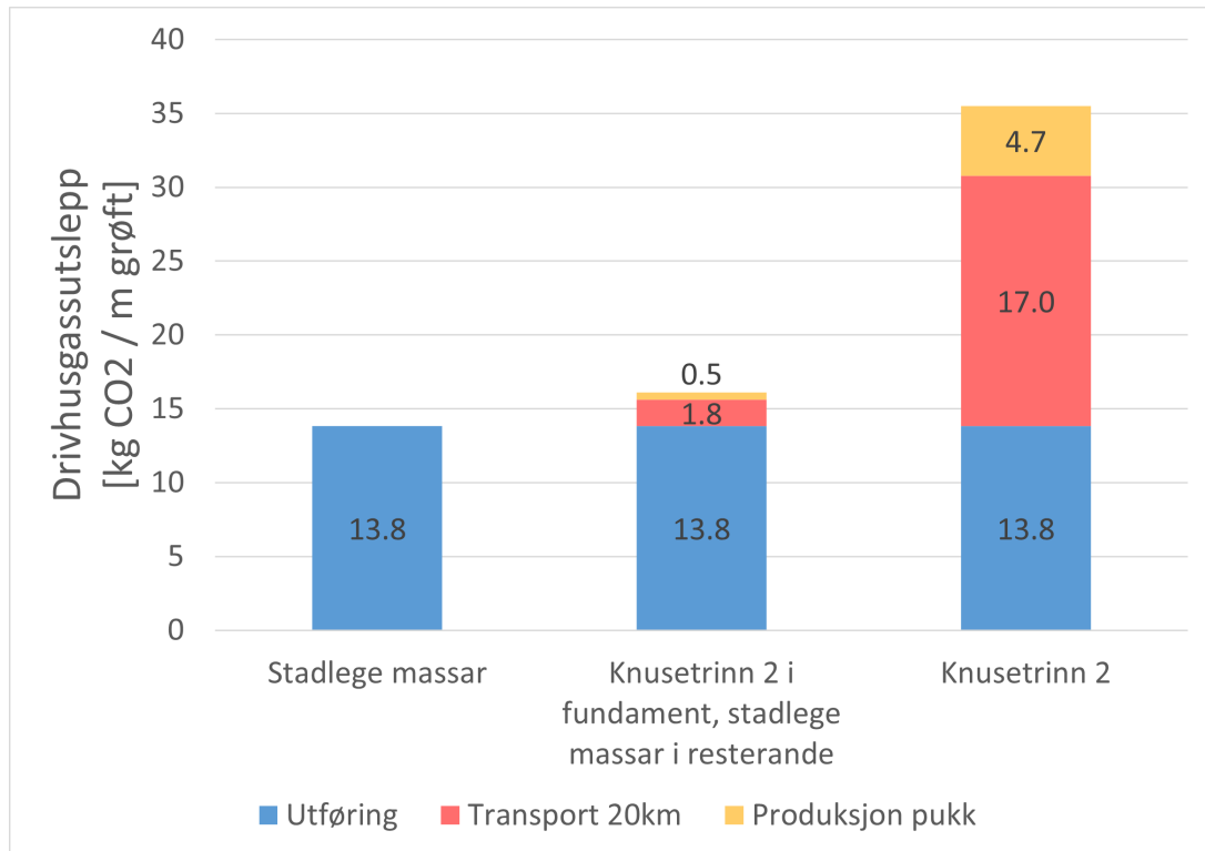
Figur 3.6: CO 2 -utslepp for produksjon av ulike massar i røyersona for fleirrøysgrøfter utanom veg.
