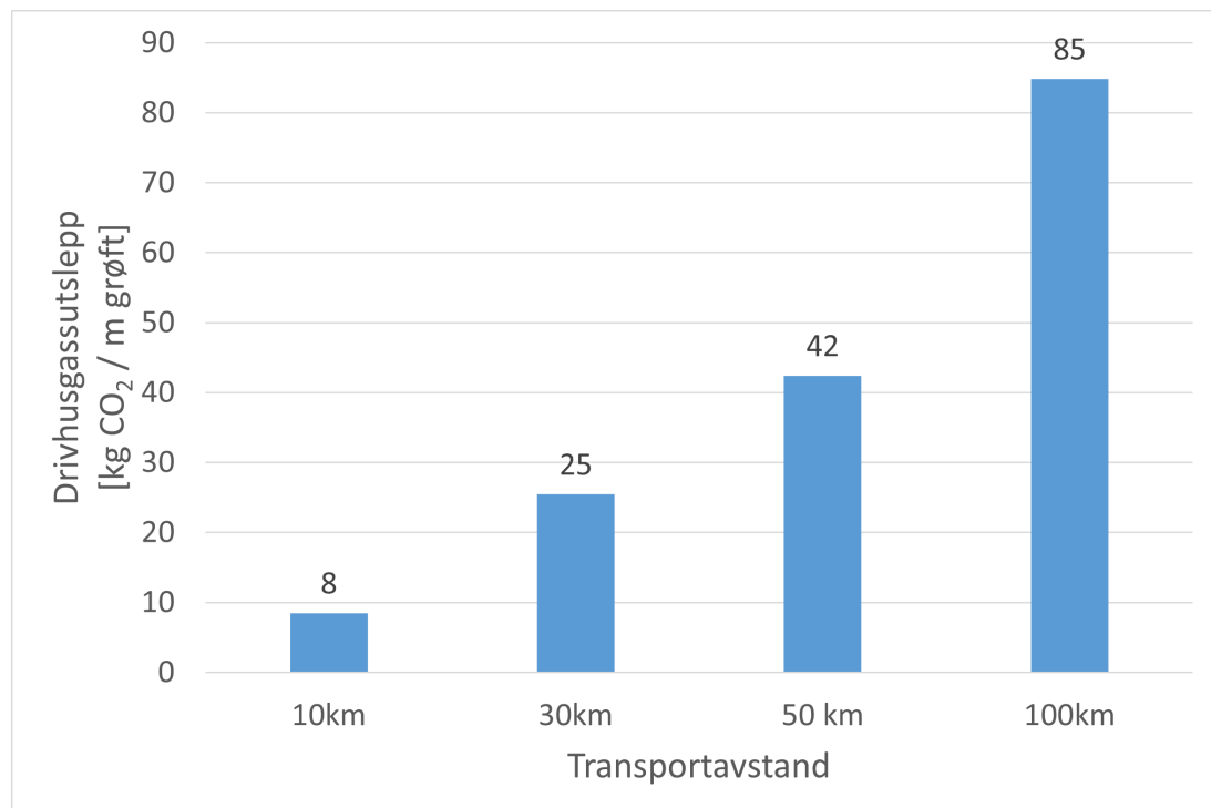
Figur 3.9: Miljøpåverknadar for ulike transportavstandar for fleirøyrgrøfter.
