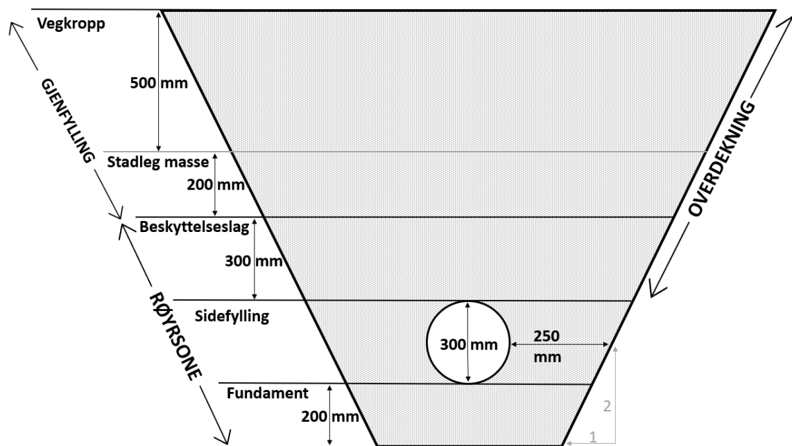
Figur 2.2: Utgangspunkt for analyse til eitrørgrøfter med røyr diameter 300 millimeter. Røyrstorleik og mål i røyrsona er likt for alle variablar av grøfta, med unntak av grøftehelling og gjenfylling.
