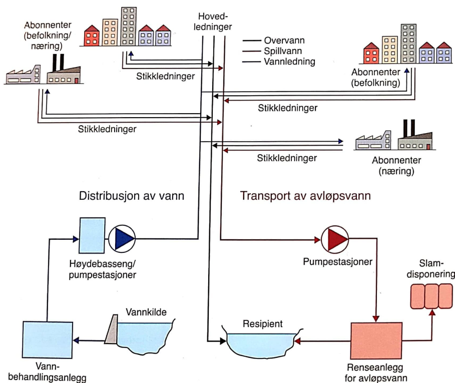
Figur 1.1: Korleis det norske vass-, avløps- og overvassnettet heng saman. (Norsk Vann, 2014)
