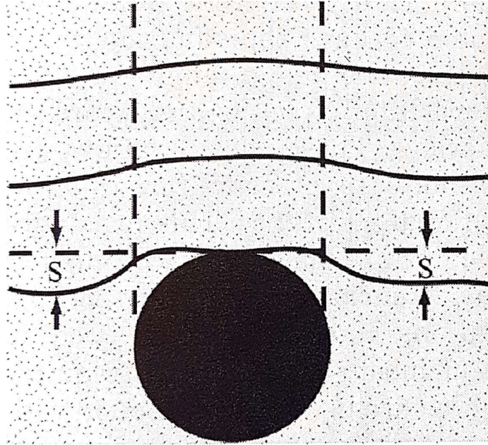
Figur 1.3: Korleis setningane i jorda blir om ein har eit stivt røyr. I sidefyllinga vil jorda synke noko saman, medan det stive røynet vil halde på same form. Her representerer S kor mykje sidefyllinga vil sette seg. (Moser, 2001)
