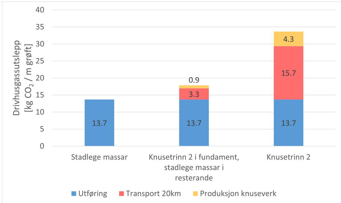
Figur 3.4: CO 2 -utslepp for produksjon av ulike massar i røyrsona for eitrøyrgrøfter med røyrdimensjon 600 millimeter utanom veg.
