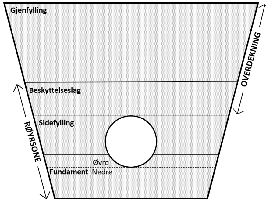
Figur 1.6: Oppbygging av ei røyrgroft med eit røyre.
