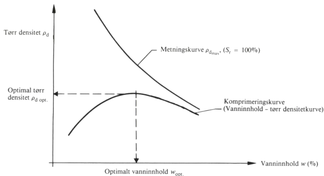
Figur 1.15: Forholdet mellom tørr densitet og vassinnhald for ein gjeven jordart og eit gjeven komprimeringsarbeid. (Aarhaug, 1984) Figur 1.32
