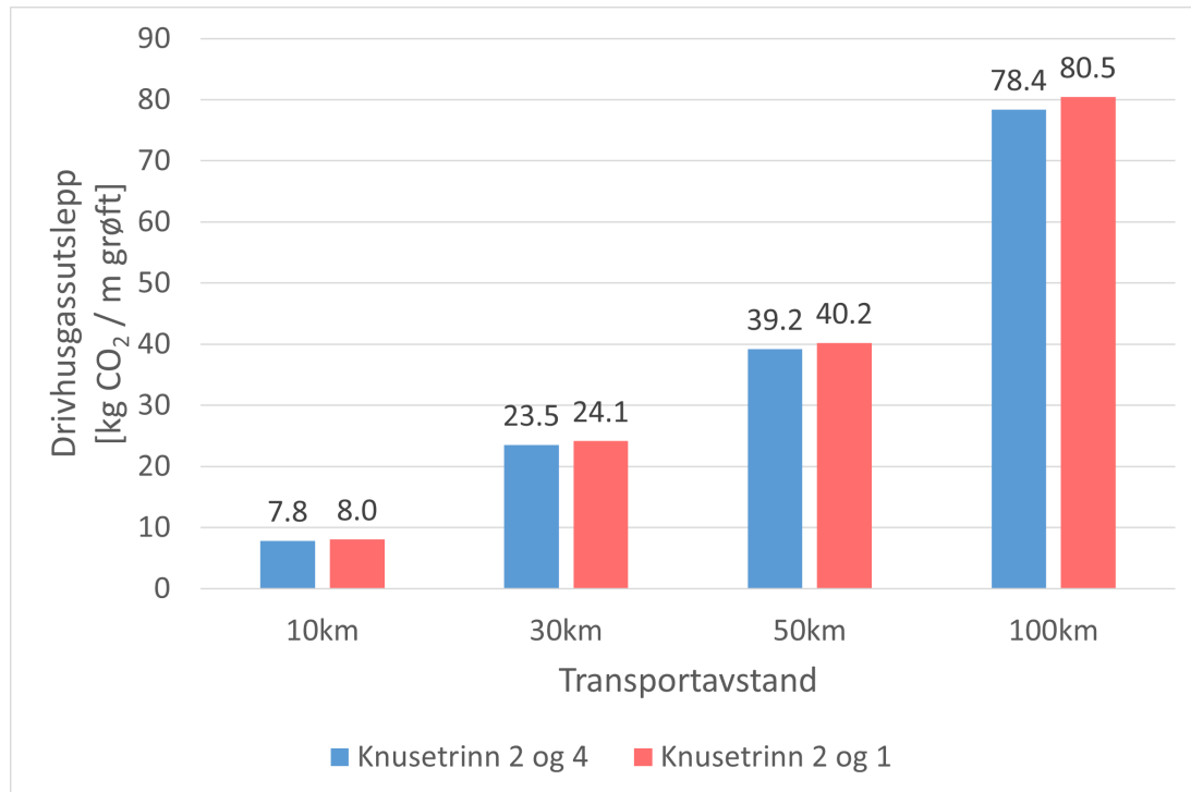
Figur 3.8: Miljøpåverknadar for ulike transportavstandar for eitrøyrgrøfter med røyrdimensjon 600 millimeter.
