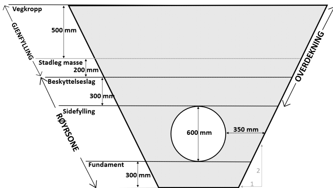
Figur 2.3: Utgangspunkt for analysa til eitrøyrgrøfter med røyr diameter 600 millimeter. Røyrstorleik og mål i røyrsona er likt for alle variablar av grøfta, med unntak av grøftehelling og gjenfylling.
