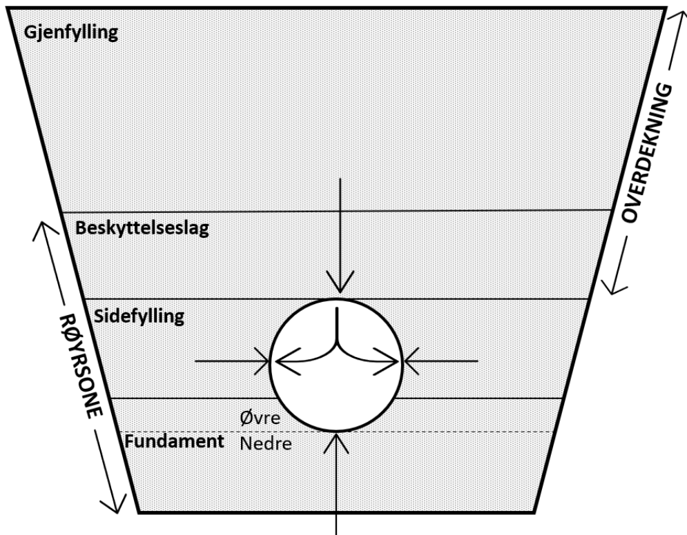
Figur 1.4: Korleis laster frå jorda verkar på fleksible røyr. Det verkar både horisontale og vertikale krefter på røyrret. Korrekt oppbyggnad av sidefylling er derfor viktig for å unngå deformering av røyrret. Figur utforma etter inspirasjon frå Moser (2001).
