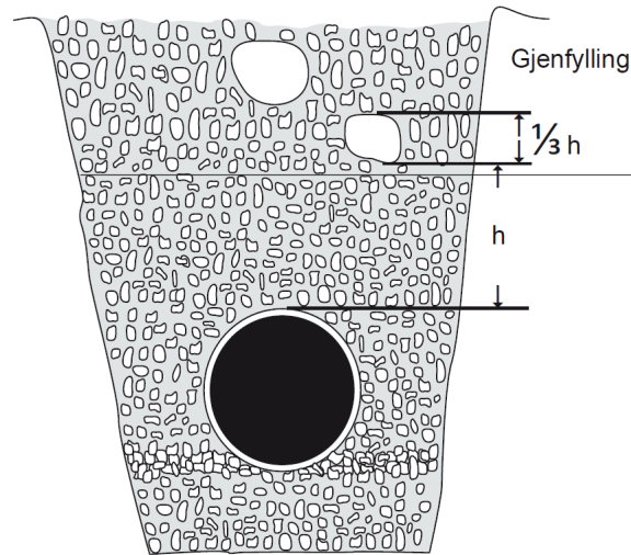
Figur 1.14: Plastrøyrproduzentane sitt krav til største kornstorleik i gjenfyllinga. (NPG, 2018)
