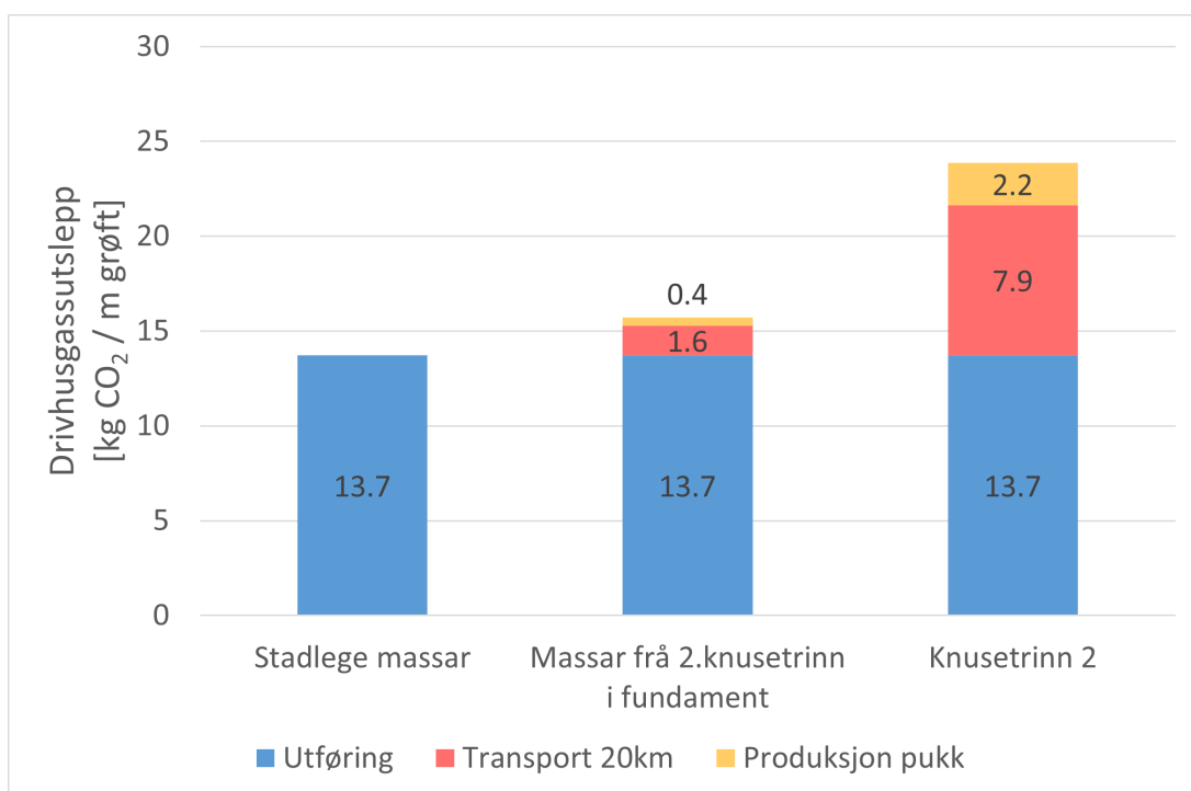
Figur 3.2: CO 2 -utslepp frå heile livsløpet for eit røyrsgrøft utanom veg med overdekning ein meter utanom veg.
