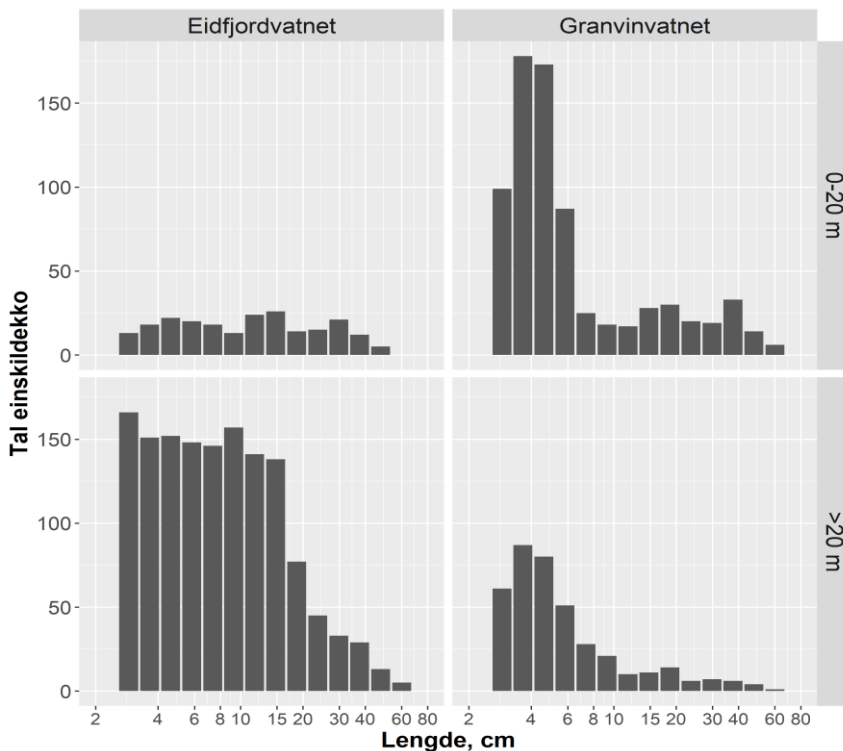
Figur 25. Tal einskildekkko (y-aksen) og lengdefordeling (x-aksen) for Eidfjordvatnet og Granvinsvatnet. Estimert frå ekkodata samla inn oktober 2019.
