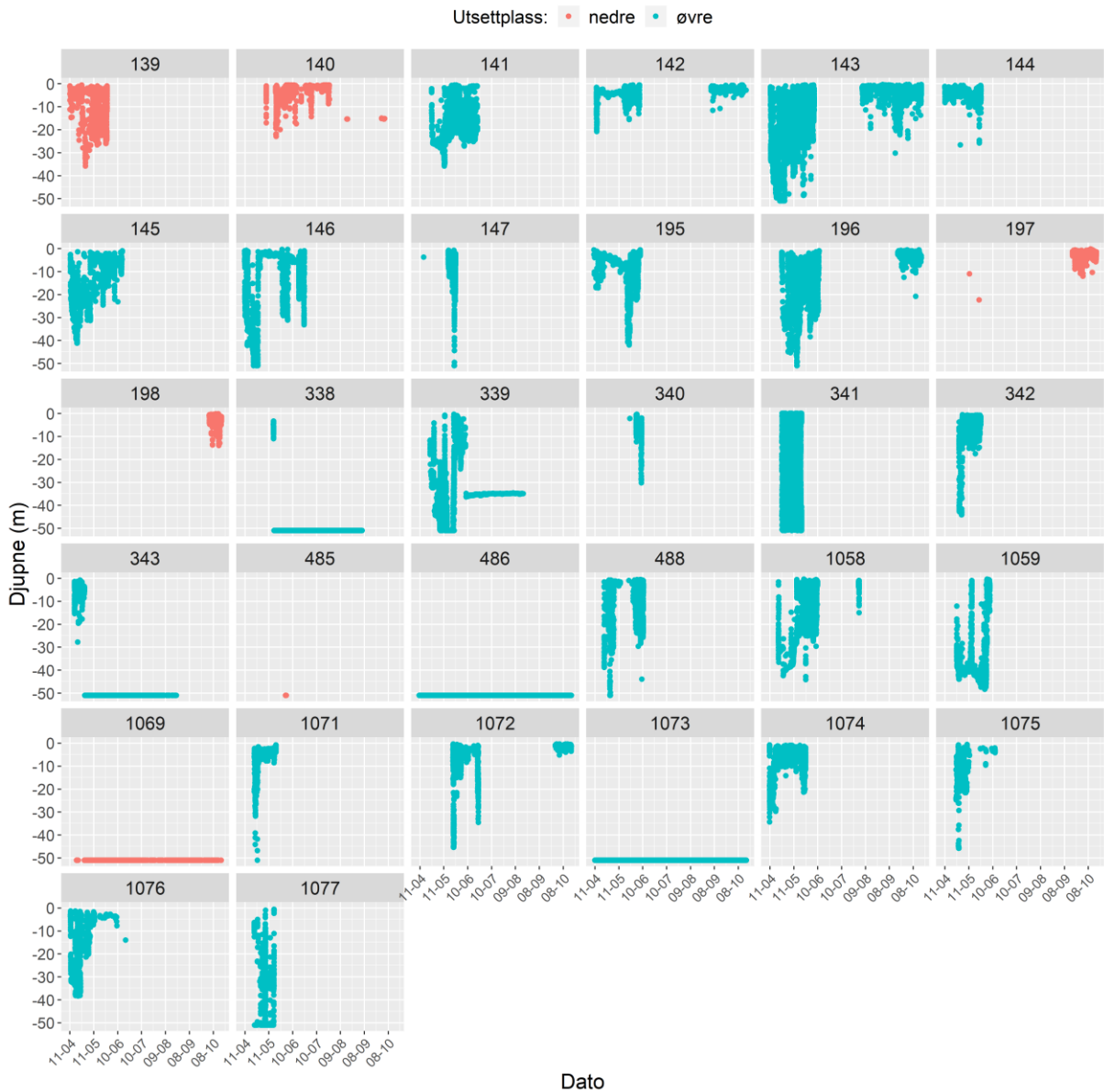
Figur 14. Djupnebruk til akustisk merka aure i Eidfjordvatnet. Aurane er delt i to grupper, blå plott symboliserer aure sett ut i Bjoreio (innlaupselv) og oransje plott symboliserer aurar sett ut i Eio (Utlaupeelv) (ID i figurpanela).
