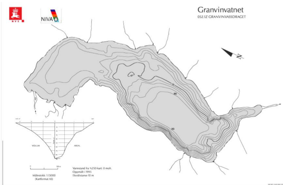
Figur 4. Djupekart over Granvinvatnet, henta frå (NVE-atlas.no)
