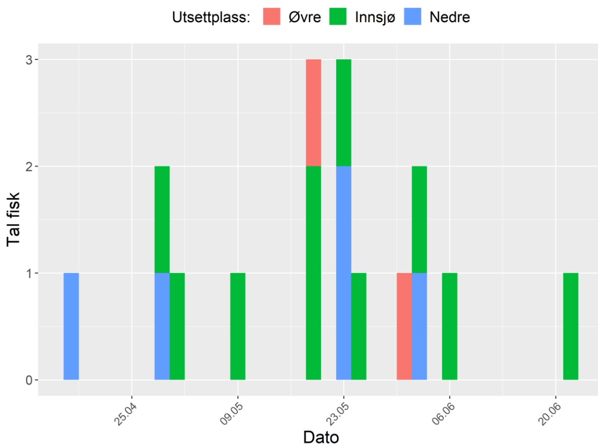
Figur 9. Utvandringstidspunkt frå ferskvatn til fjord, Granvinsvassdraget. Aure satt ut i Granvinselva er illustrert med blå søyler, Aure satt ut i Granvinsvatnet illustrert med grønne søyler og aure satt ut i Storelvi er illustrert med oransje. Tal aure detektert (Y-aksen), dato detektert (x-aksen).
