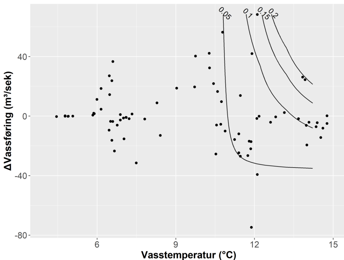
Figur 12. Predikert døgnleg sannsyn for aureutvandring frå Eidfjordvassdraget, forklart gjennom \Delta vassføring (Y-aksen) og vass temperatur (X-aksen). Sannsyna er framstilt som konturlinjer der dei respektive sannsynsverdiane er gjeve som tal øvst på linjene. Estimata kjem frå den utvalde modellen som er rapportert i Tabell 7 .
