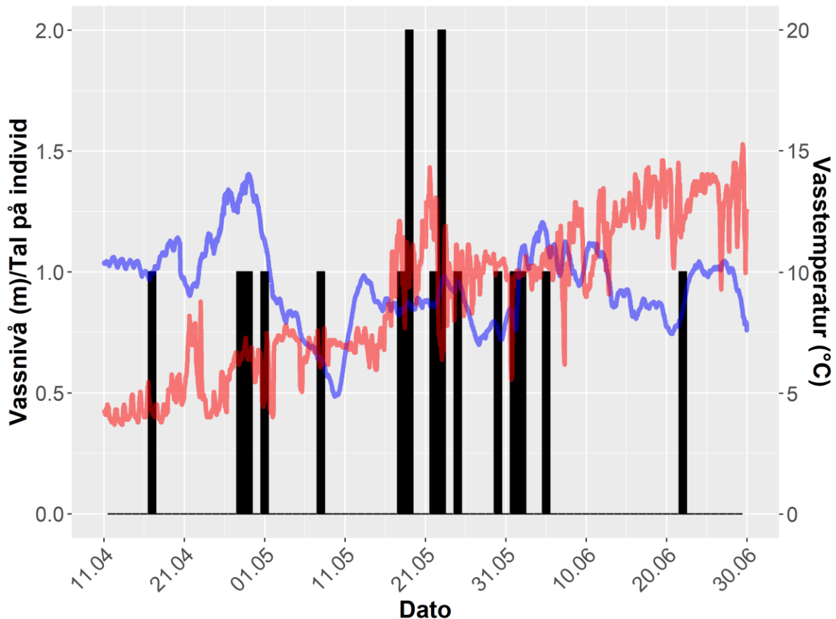
Figur 11. Utvandringstidspunkt frå ferskvatn til fjord, Granvinsvassdraget. Utvandring av aurar presentert som svarte søyler, med overliggende vasstemperatur og vassnivå for perioden 11. april – 30. juni 2019. Blå linje syner vassnivå, raud linje syner vasstemperatur.
