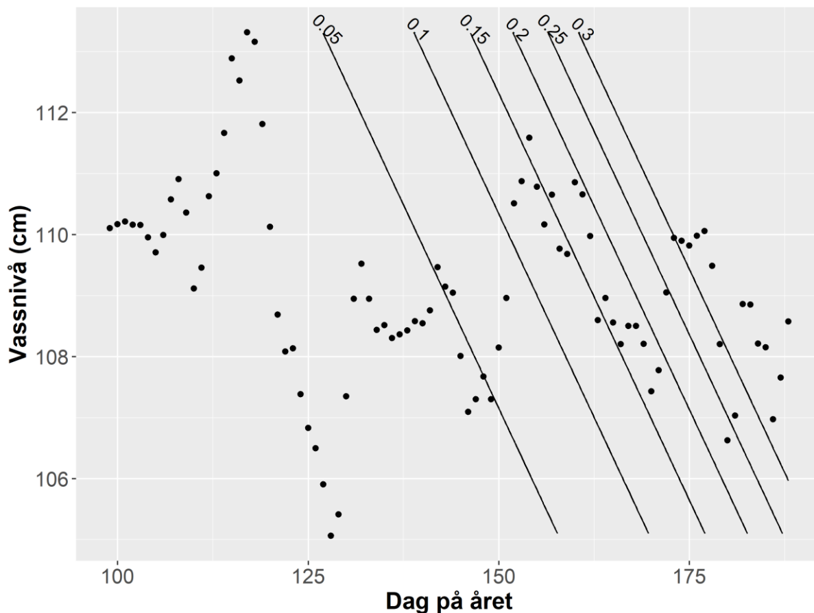
Figur 13. Prediktert døgnetlig sannsyn for aureutvandring frå Granvinsvassdraget, forklart gjennom Vassnivå (cm) (Y-aksen) og Dag på året (x-aksen). Sannsyna er framstilt som konturlinjer der dei respektive sannsynsverdiene er gjeve som tal øvst på linjene. Dag på året 150 = 29. mai 2019. Estimata kjem frå den utvalde modellen som er rapportert i Tabell 9 .
