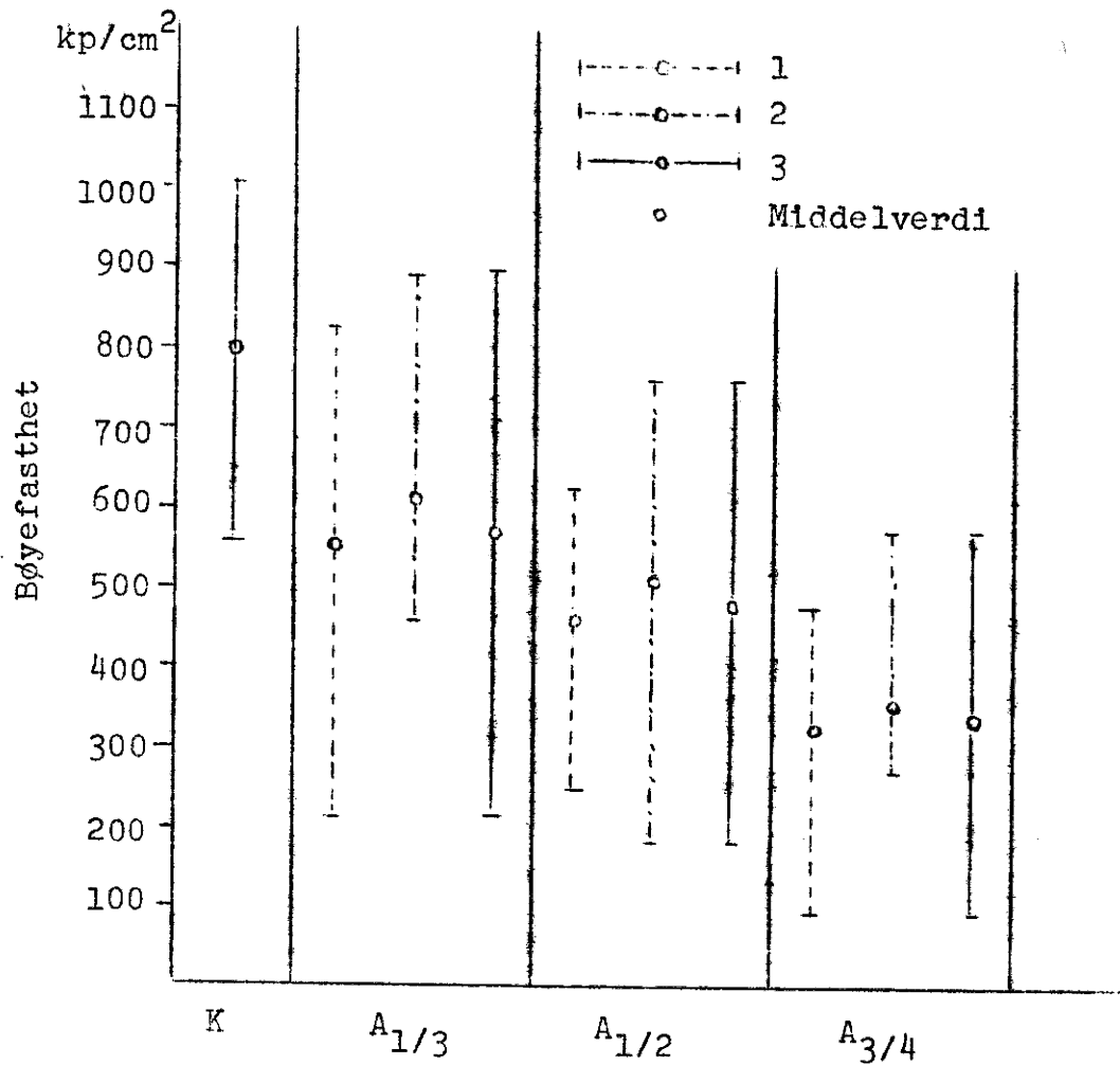
Figur 2. Bøyefasthetens variasjon med kvistinnhold hos gran. Middelverdier og spredning (etter KUCERA 1970).
