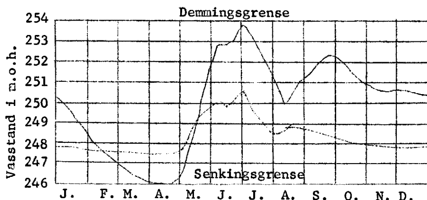
Fig. 33, viser vasstandene i regulert sjø i 1951, hel linje. Streket linje viser vasstandene som de var i uregulert sjø.
