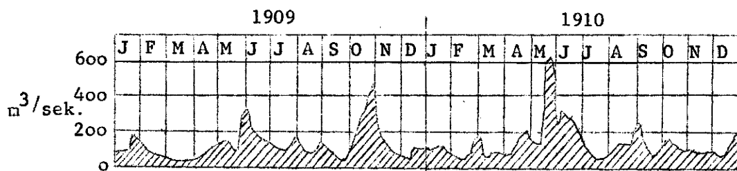
Vassføring i Sira ved Lundevatn
