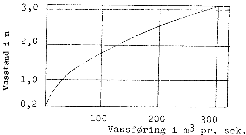
Fig. 35 Vassføringskurve for vassmerke: Tunhovd, Numedalslågen.
