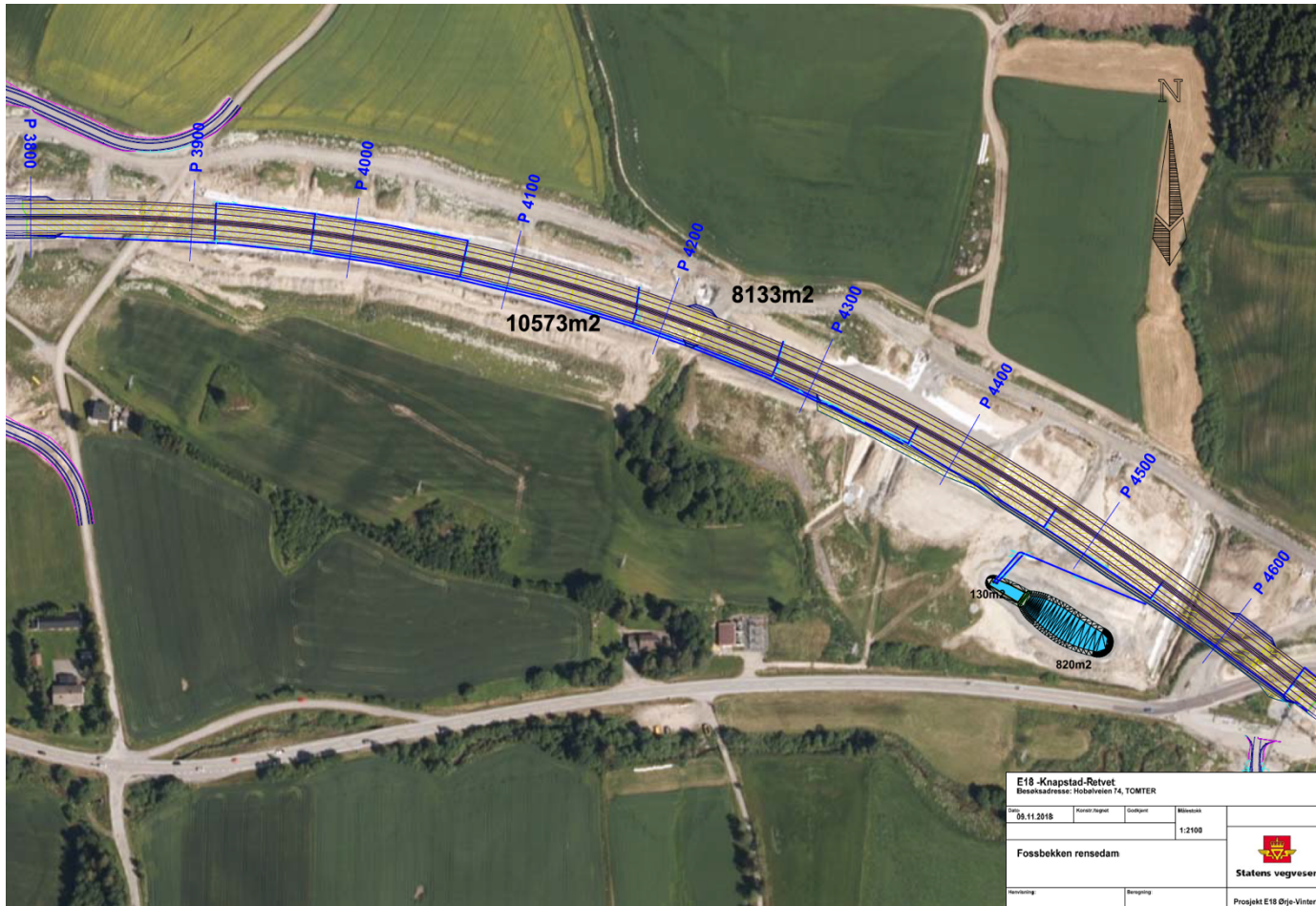
Figur 30: Plankart fra Statens vegvesen over Fossbekken rensedam, med arealinformasjon om rensedammens vannvolum, areal avrenning og beliggenhet.
