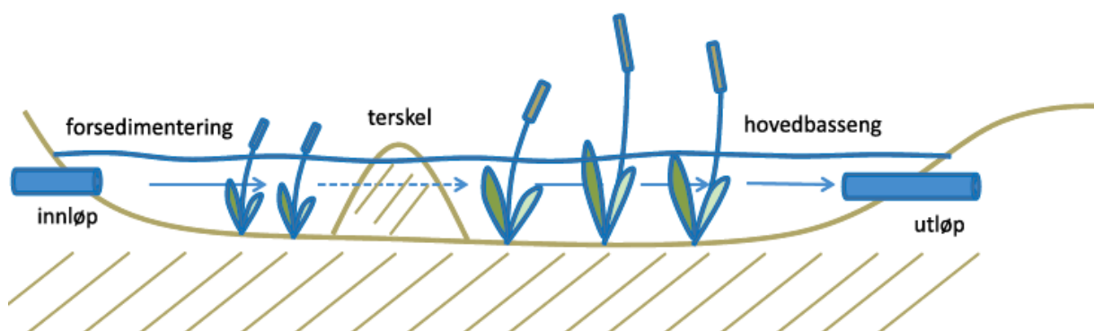
Figur 4: Illustrasjon av rensedam med vått overvannsbasseng. Forsedimentasjonsbassenget og hovedsedimentasjonsbassenget er avskilt med en terskel (ofte bygget i sten eller betong). Innløp fra Innløpskum til forsedimentasjonsbassenget, utløp til utløpskummen i hovedsedimentasjonsbassenget. Illustrasjon er hentet fra (Meland et al., 2014).
