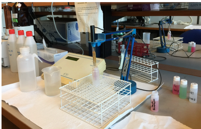
Figur 11: pH-meter, bilde viser pH måling av vannprøver. Illustrasjon av glasselektrode er hentet fra (Miljøolare, u.å).
