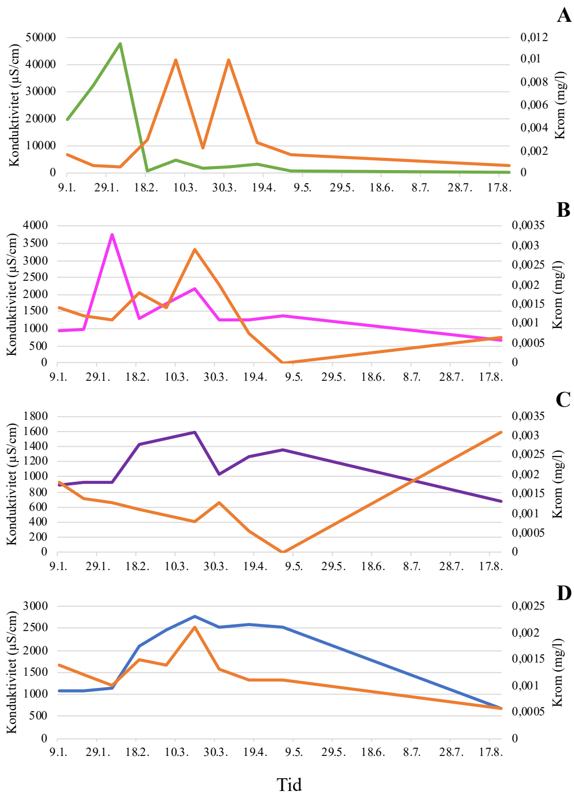
Figur 15: Krom og konduktivitet vist i tidsperioden 09.01.2019 til 17.08.2019 i innløpskummen (A), Innløpet til rensedammen (B), utløpet til rensedammen (C) og utløpskummen (D) til Fossbekken rensedam. Tid er angitt på x-aksen, konduktivitet i \mu\text{S}/\text{cm} på y-aksen og krom i mg/l på sekundær-aksen.
