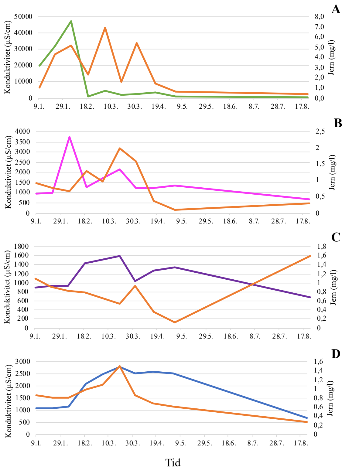
Figur 16: Jern og konduktivitet vist i tidsperioden 09.01.2019 til 17.08.2019 i innløpskummen (A), innløpet til rensedammen (B), utløpet til rensedammen (C) og utløpskummen (D) til Fossbekken rensedam. Tid er vist på x-aksen, konduktivitet i \mu\text{S/cm} på y-aksen og jern i \text{mg/l} på sekundær-aksen.
