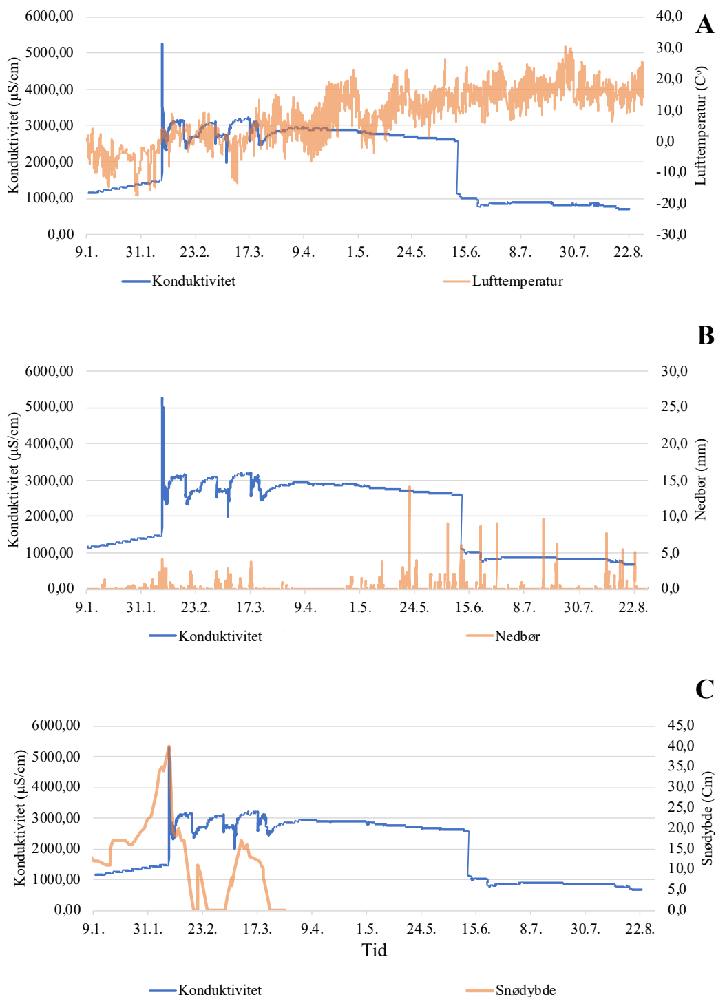
Figur 15: Konduktivitet og metrologiske data registrert for utløpskummen til Fossbekken rensedam, i analyseperioden 9. januar 2019 til 22. august 2019. Konduktivitet ble registrert hver time gjennom hele analyseperioden. Metrologiske data er hentet fra BIOKLIM værstasjon i Ås (universitet, 2020). Metrologiske data i form av nedbør, lufttemperatur og snødybde er fremvist i figuren sammen med logget konduktivitet. Analyseperioden er angitt som x-akse, konduktivitet i \mu\text{S/cm} på y-aksen og metrologisk data på sekundær -aksen.
