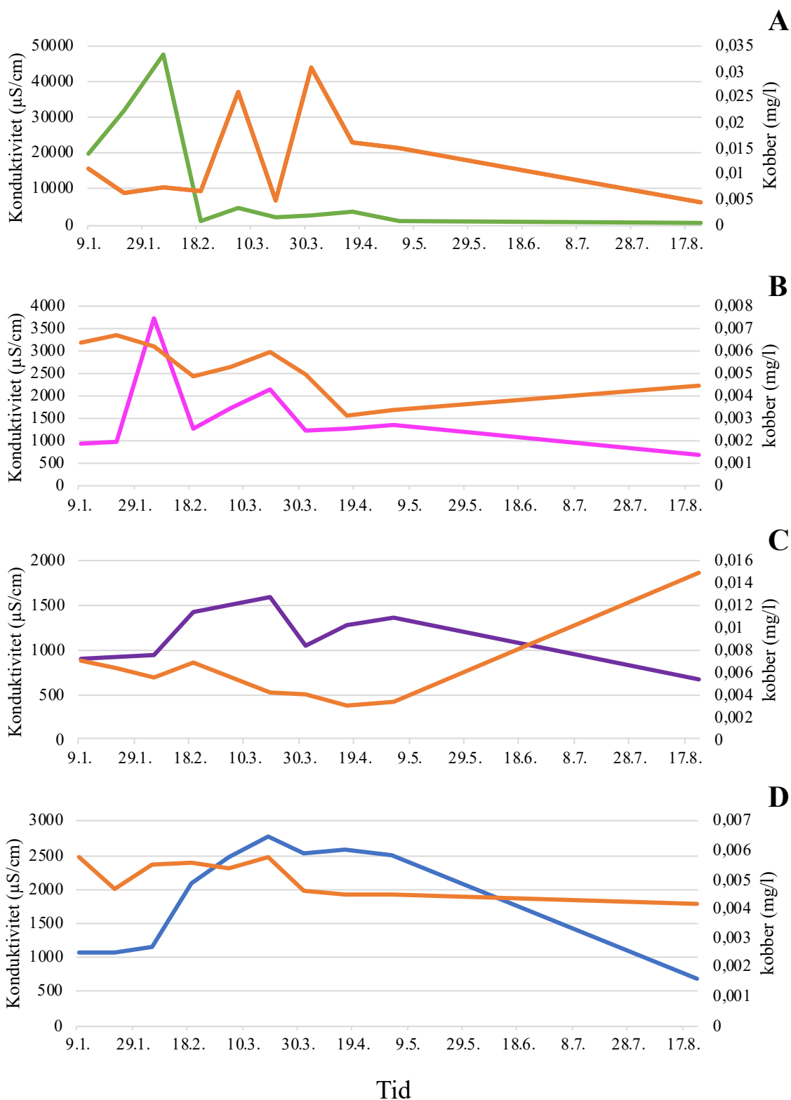
Figur 14: Kobber og konduktivitet vist i tidsperioden 09.01.2019 til 17.08.2019 i Innløpskummen (A), innløpet til rensedammen (B), utløpet til rensedammen (C) og utløpskummen (D) til Fossbekken rensedam. Tid er angitt på x-aksen, konduktivitet i \mu\text{S}/\text{cm} på y-aksen og kobber i \text{mg}/\text{l} på sekundær-aksen.
