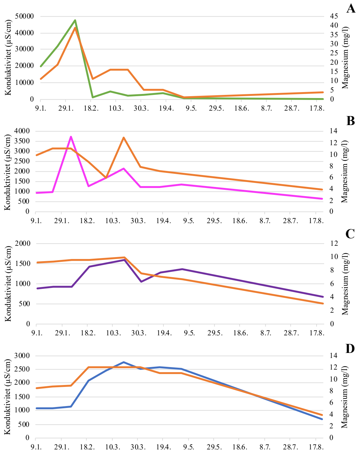
Figur 10: Magnesium og konduktivitet vist i tidsperioden 09.01.2019 til 17.08.2019 i innløpskummen (A), innløpet til rensedammen (B), Utløpet til rensedammen (C) og utløpskummen (D) til Fossbekken rensedam. Tid er vist på x-aksen, konduktivitet i \mu\text{S/cm} og y-aksen og magnesium i \text{mg/l} på sekundær-aksen.
