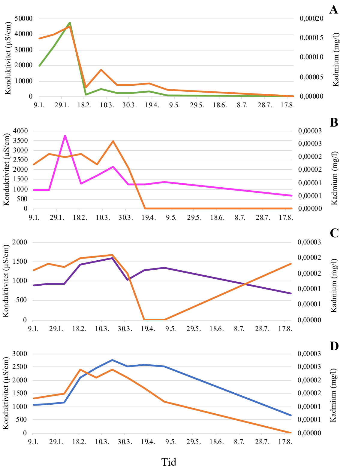
Figur 13: Kadmium og konduktivitet vist i tidsperioden 09.01.2019 til 17.08.2019 i innløpskummen (A), innløpet til rensedammen (B), Utløpet til rensedammen (C) og utløpskummen (D) til Fossbekken rensedam. Tid er vist på x-aksen, konduktivitet i \mu\text{S/cm} og y-aksen og kadmium i \text{mg/l} på sekundær-aksen.
