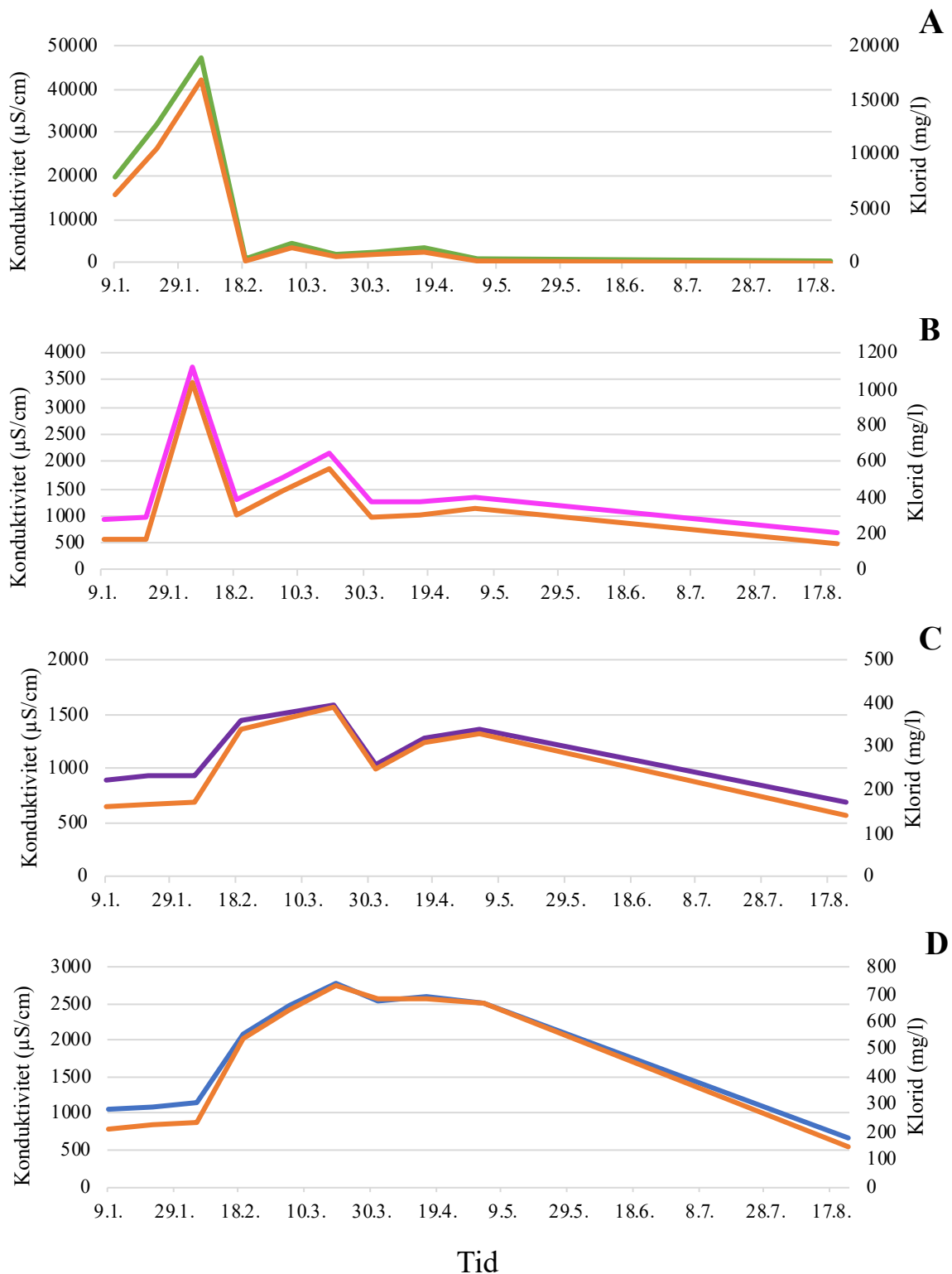
Figur 7: Klorid og konduktivitet i \text{mg/l} i innløpskummen (A), Innløpet til rensedammen (B), Utløpet til rensedammen (C) og i utløpskummen (D) til Fossbekken rensedam. Klorid og konduktivitet er fremvist i tidsperioden 09.01.2019 til 17.08.2019. Tid er angitt på x-aksen, konduktivitet i \mu\text{S/cm} på y-aksen og klorid i \text{mg/l} på sekundær-aksen.
