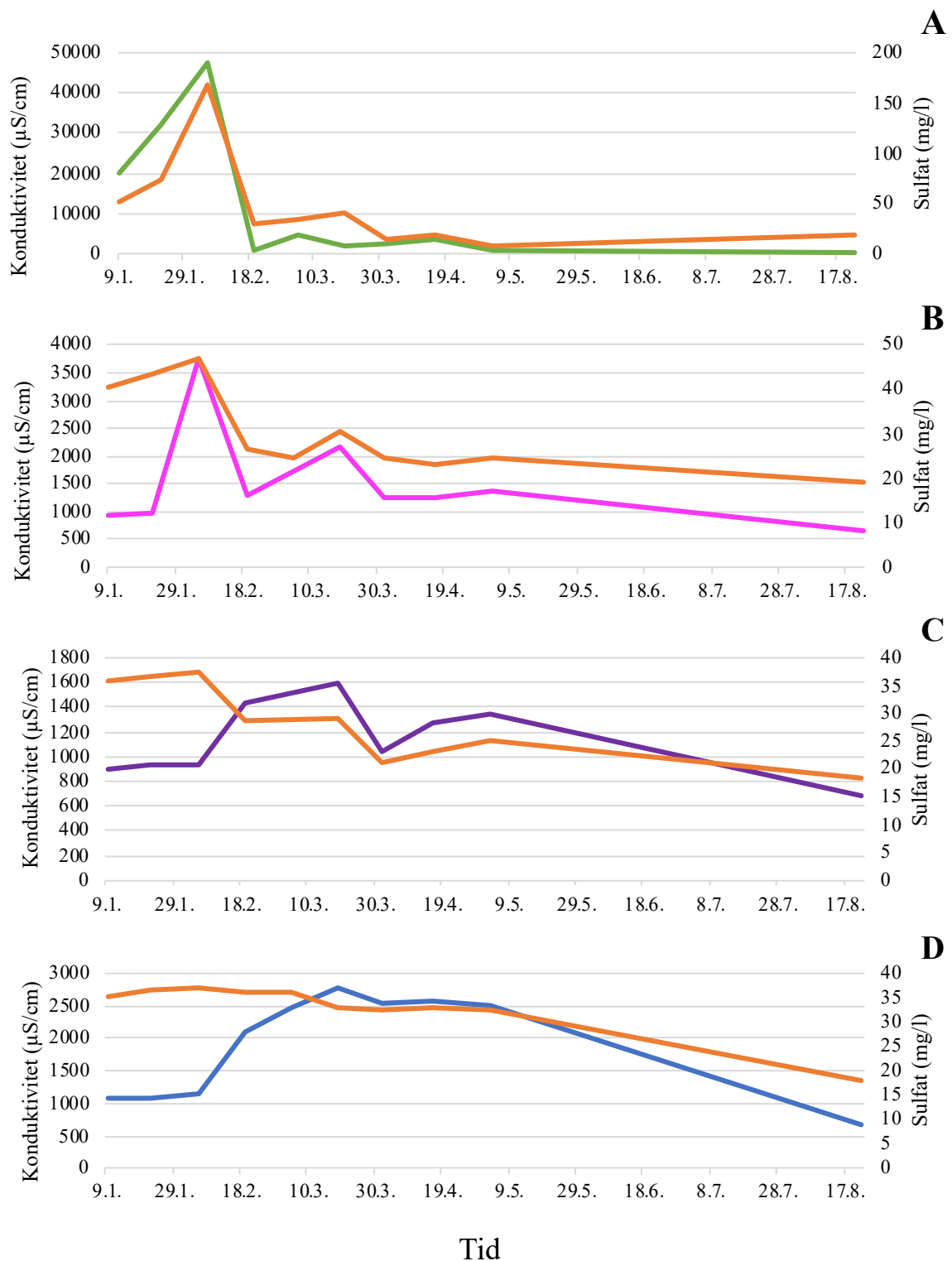
Figur 8: Sulfat og konduktivitet er fremvist i tidsperioden 09.01.2019 til 17.08.2019 i Innløpskummen (A), innløpet til rensedammen (B), utløpet til rensedammen (C) og utløpskummen (D) til Fossbekken rensedam. Tid er angitt på x-aksen, konduktivitet i \mu\text{S/cm} på y-aksen og sulfat i \text{mg/l} på sekundær-aksen.
