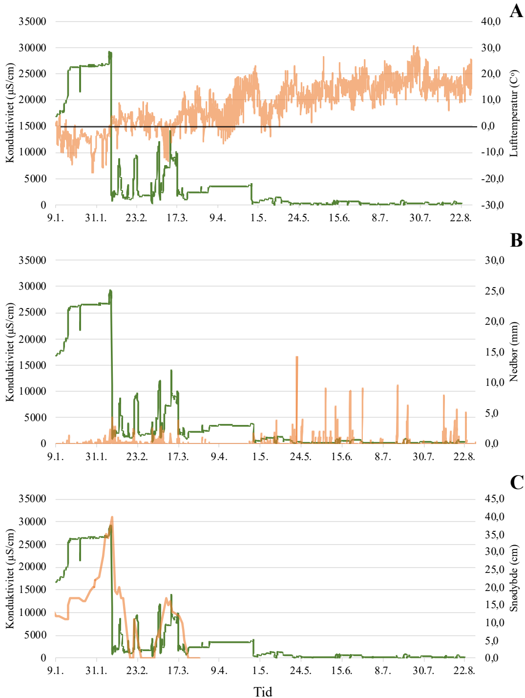
Figur 13: Konduktivitet (temperaturjustert) for innløpskummen til Fossbekken rensedam, i analyseperioden 9. januar 2019 til 22. august 2019. Konduktivitet og metrologiske data ble registrert hver time gjennom hele prøveperioden. Metrologiske data er hentet fra BIOKLIM værstasjon Ås (universitet, 2020). Spesifikk konduktivitet er fremvist i samsvar med metrologiske data i form av lufttemperatur (A), nedbør (B) og snødybde (C). Analyseperioden er angitt på x-aksen, spesifikk konduktivitet på y-aksen og metrologiske data på sekundær-aksen.
