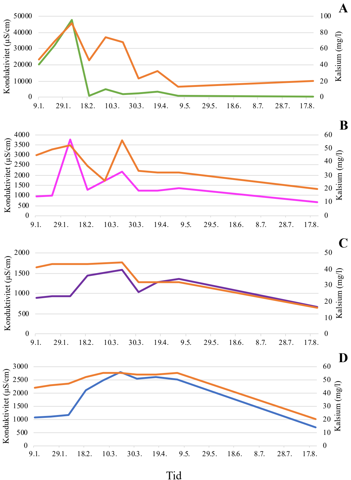
Figur 9: Kalsium og konduktivitet vist i tidsperioden 09.01.2019 til 17.08.2019 i innløpskummen (A), innløpet til rensedammen (B), Utløpet til rensedammen (C) og utløpskummen (D) til Fossbekken rensedam. Tid er vist på x-aksen, konduktivitet i \mu\text{S/cm} og y-aksen og kalsium i \text{mg/l} på sekundær-aksen.
