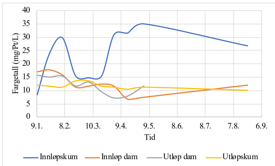
Figur 4: Fargetall (mg/Pt/L) i Fossbekken rensedam innløp og utløp, innløpskum og utløpskum i perioden 09.01.2019 til 22.08.2019. Tid er vist på x-aksen.
