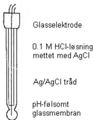
Figur 11: pH-meter, bilde viser pH måling av vannprøver. Illustrasjon av glasselektrode er hentet fra (Miljøolare, u.å).
