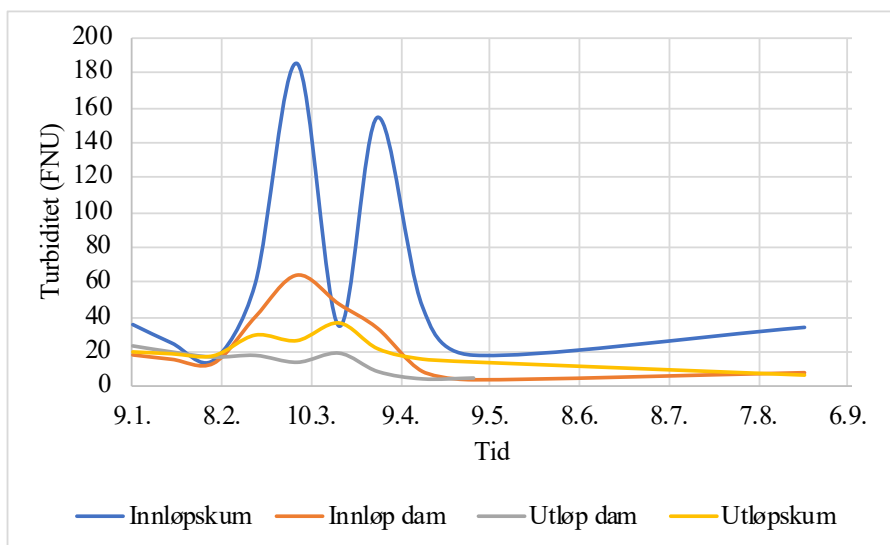
Figur 3: Turbiditet Fossbekken, innløpskum, utløpskum, innløpet til rensedammen og utløpet til rensedammen i perioden 09.01.2019 til 22.08.2019. Tid er angitt på x-aksen (dato) og turbiditet på y-aksen.
