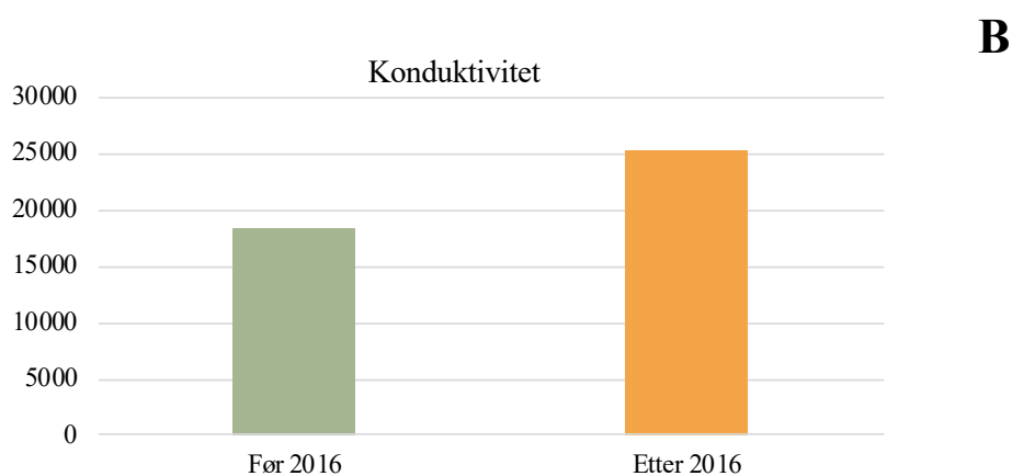
Figur 18: Gjennomsnittlige verdier av vannanalyser i Fossbekken før og etter etablering og drift av Fossbekken rensedam. Det ble benyttet gjennomsnittlige verdier av vannanalyser samlet i overvannet til Fossbekken. Før drift er gjennomsnitt av data fra 2014-2016 og etter drift er gjennomsnitt fra 2016-2020.
