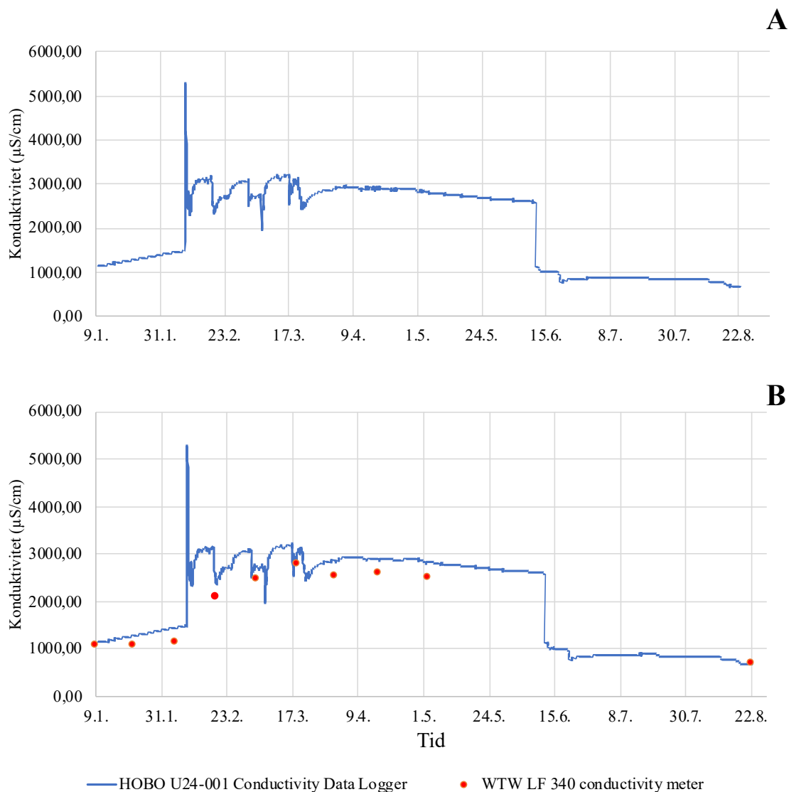
Figur 14: Konduktivitet registrert for utløpskummen til Fossbekken rensedam, i analyseperioden 9. januar 2019 til 22. august 2019. Konduktivitet ble registrert hver time gjennom analyseperioden med HOBO konduktivitetslogger, vist i figur A. Figur B viser i tillegg til logget konduktivitet, feltmålinger registrert med WTW LF 340 konduktivimeter. Feltmålingene er lagt inn i figuren for å sammenligne og validere registrert konduktivitet gjennom analyseperioden. Analyseperioden er angitt på x-aksen og konduktivitet i \mu\text{S}/\text{cm} er angitt på y-aksen.
