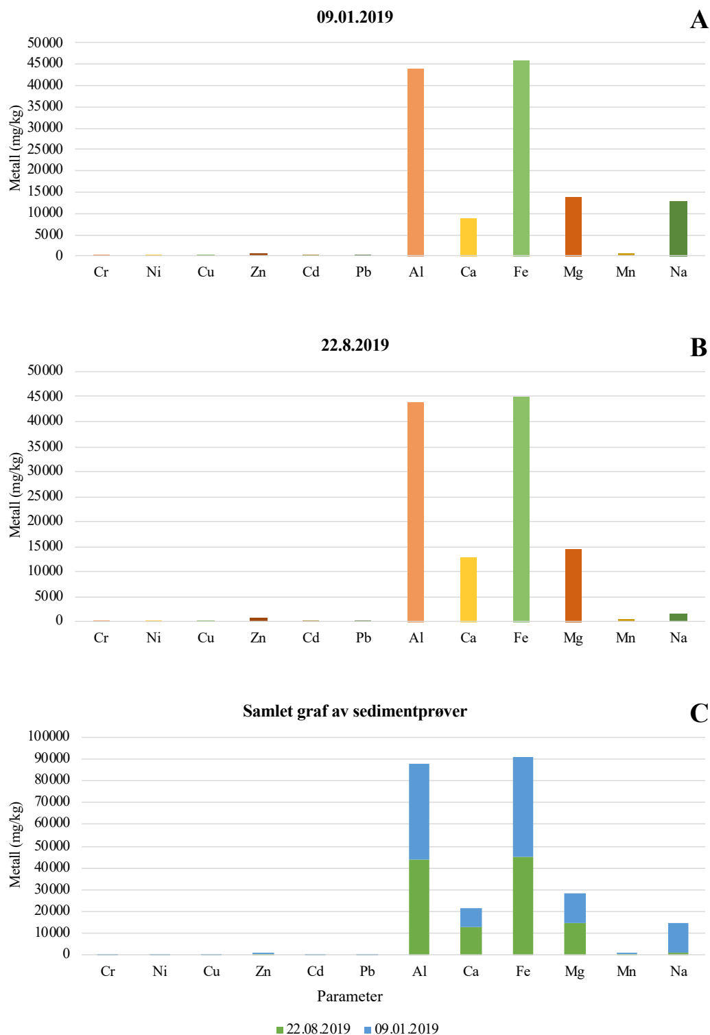
Figur 17: Sedimentprøver tatt den 9. januar.2019 vist i figur A, 22. august 2019 i figur B og sammensatt figur av de to prøvetakingsdagene i figur C. X-aksen viser parameterne analysert for i sedimentprøvene og y-aksen viser konsentrasjonen av parameterne analysert for i mg/kg.
