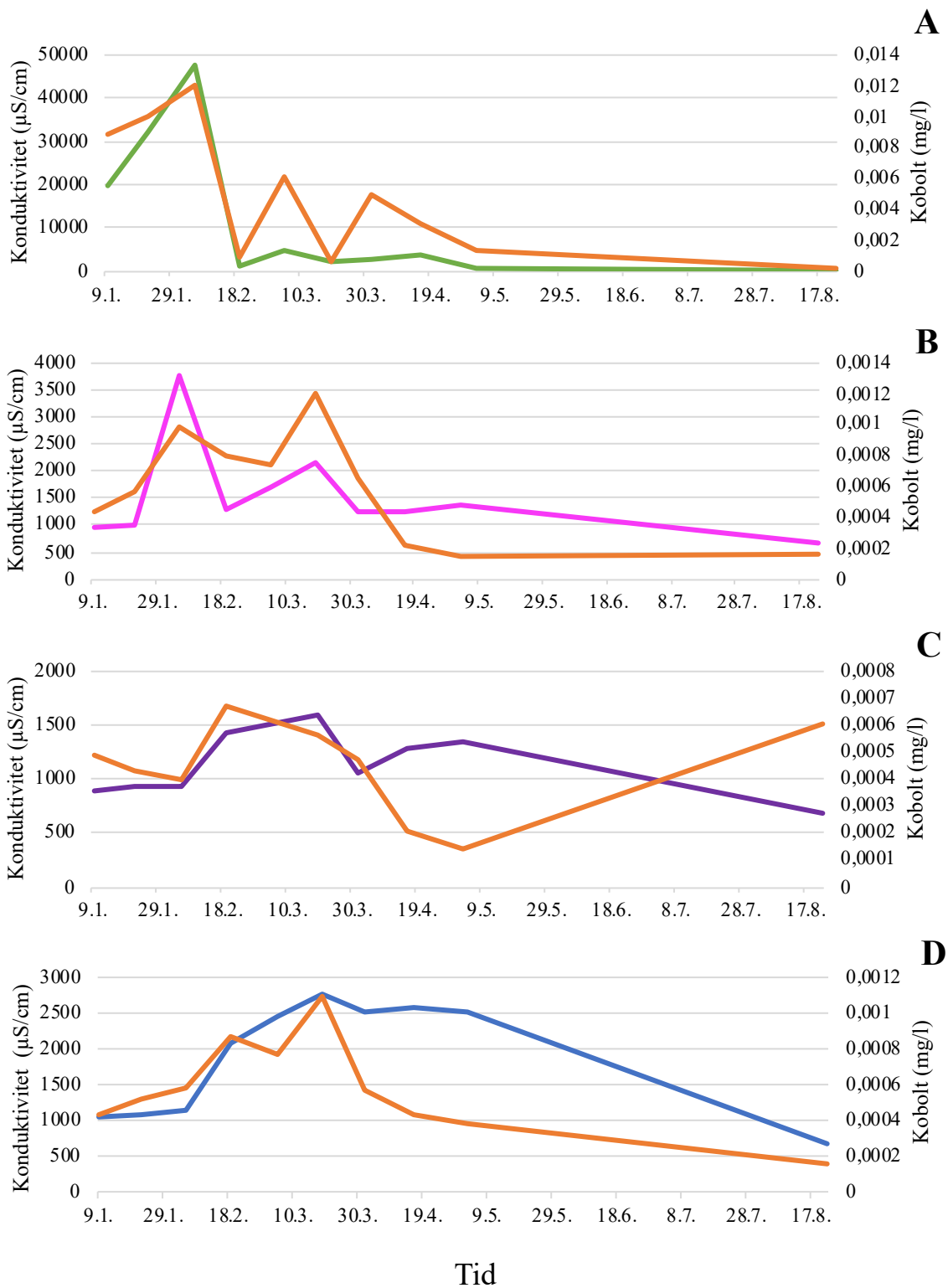
Figur 11: Kobolt og konduktivitet vist i tidsperioden 09.01.2019 til 17.08.2019 i innløpskummen (A), innløpet til rensedammen (B), utløpet til rensedammen (C) og utløpskummen (D) til Fossbekken rensedam. Tid er vist på x-aksen, konduktivitet i µS/cm på y-aksen og kobolt i mg/l på sekundær-aksen.
