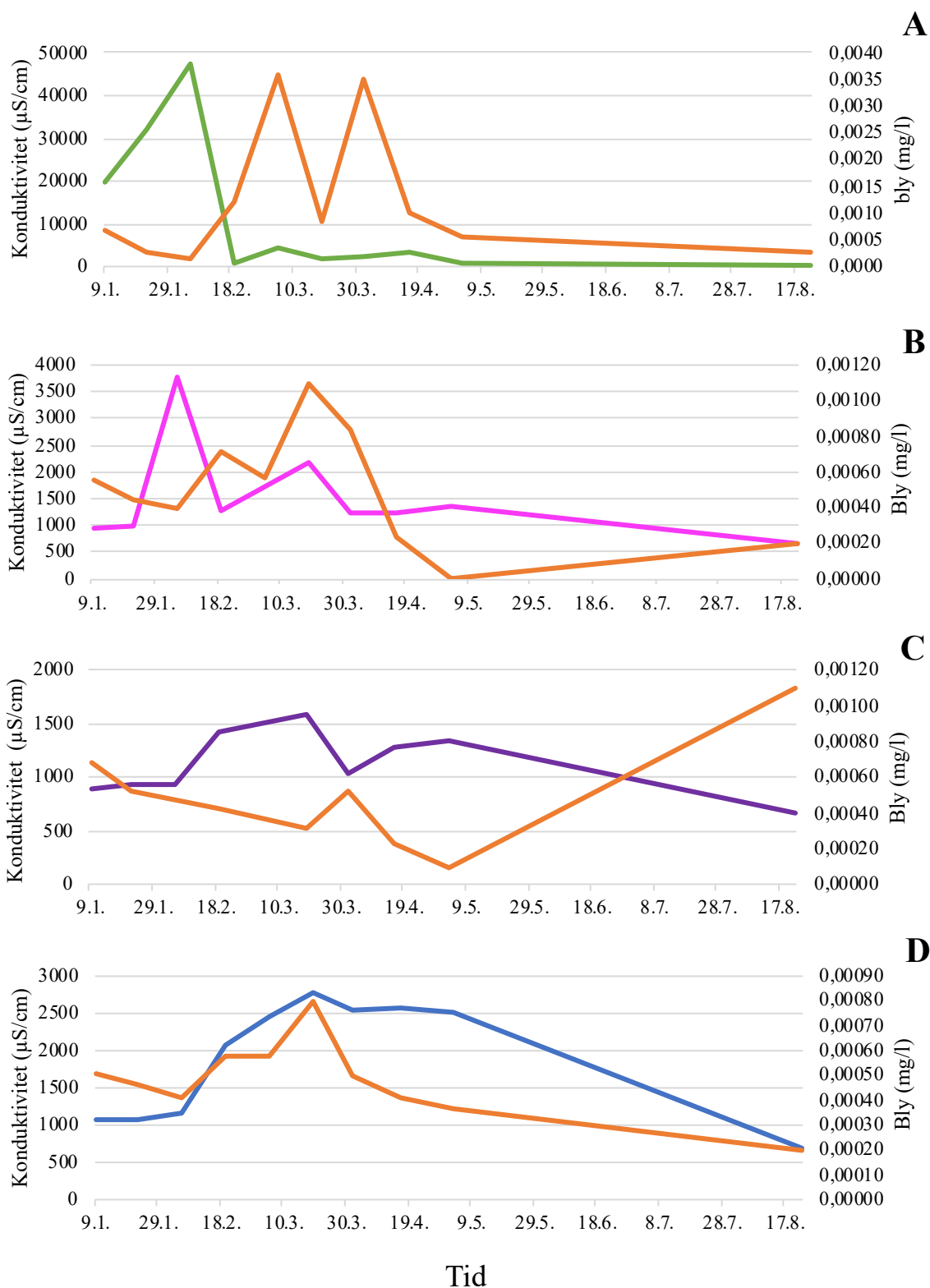
Figur 19: Bly og konduktivitet vist i tidsperioden 09.01.2019 til 17.08.2019 i innløpskummen (A), innløpet til rensedammen (B), Utløpet til rensedammen (C) og utløpskummen (D) til Fossbekken rensedam. Tid er vist på x-aksen, konduktivitet i µS/cm og y-aksen og bly i mg/l på Sekundær-aksen.
