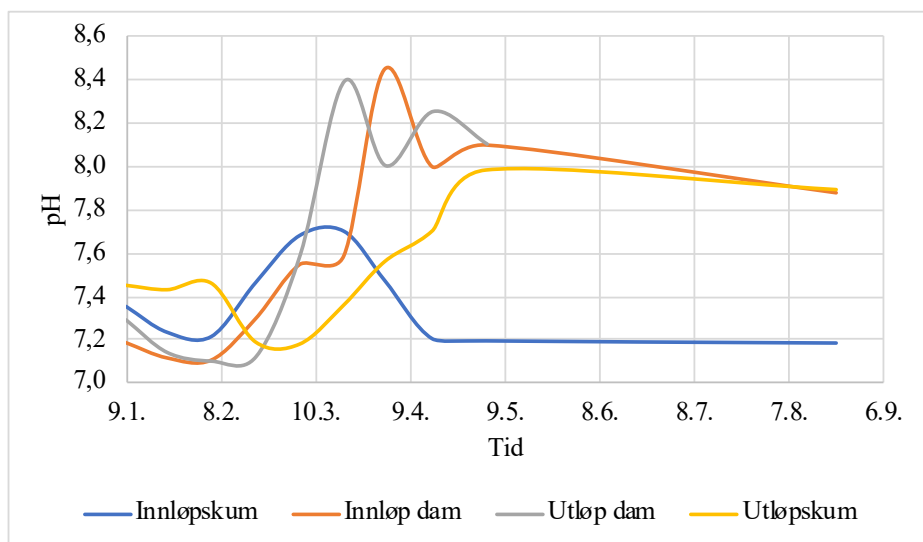
Figur 5: pH i Fossbekken rensedam innløp og utløp, innløpskum og utløpskum i perioden 09.01.2019 til 22.08.2019. Tid er vist på x-aksen.
