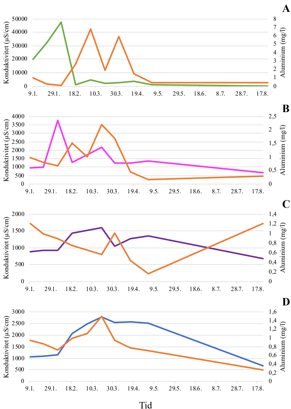
Figur 20: Aluminium og konduktivitet vist i tidsperioden 09.01.2019 til 17.08.2019 i innløpskummen (A), innløpet til rensedammen (B), Utløpet til rensedammen (C) og utløpskummen (D) til Fossbekken rensedam. Tid er vist på x-aksen, konduktivitet i \mu\text{S/cm} og y-aksen og aluminium i \text{mg/l} på Sekundær-aksen.
