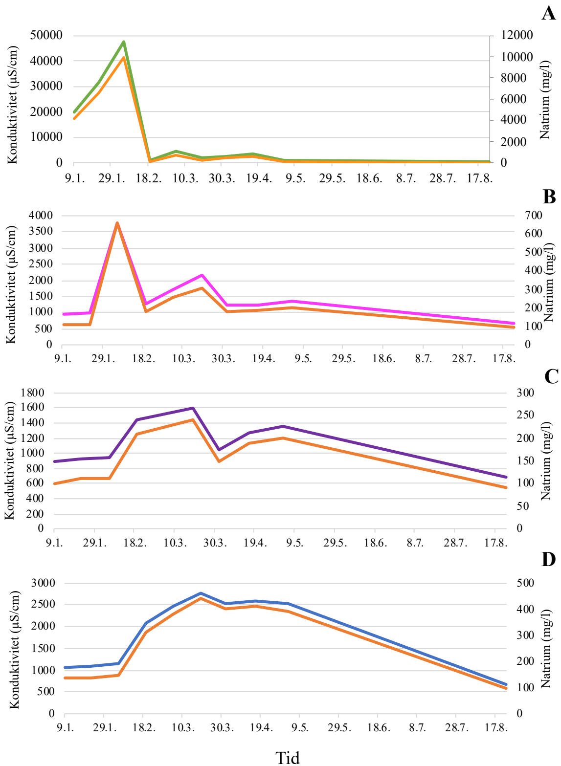
Figur 6: Natrium og konduktivitet i mg/l i innløpskummen (A), Innløpet til rensedammen (B), Utløpet til rensedammen (C) og i utløpskummen (D) til Fossbekken rensedam. Natrium og konduktivitet er fremvist i tidsperioden 09.01.2019 til 17.08.2019. Tid er angitt på x-aksen, konduktivitet i µS/cm på y-aksen og natrium i mg/l på sekundær-aksen.
