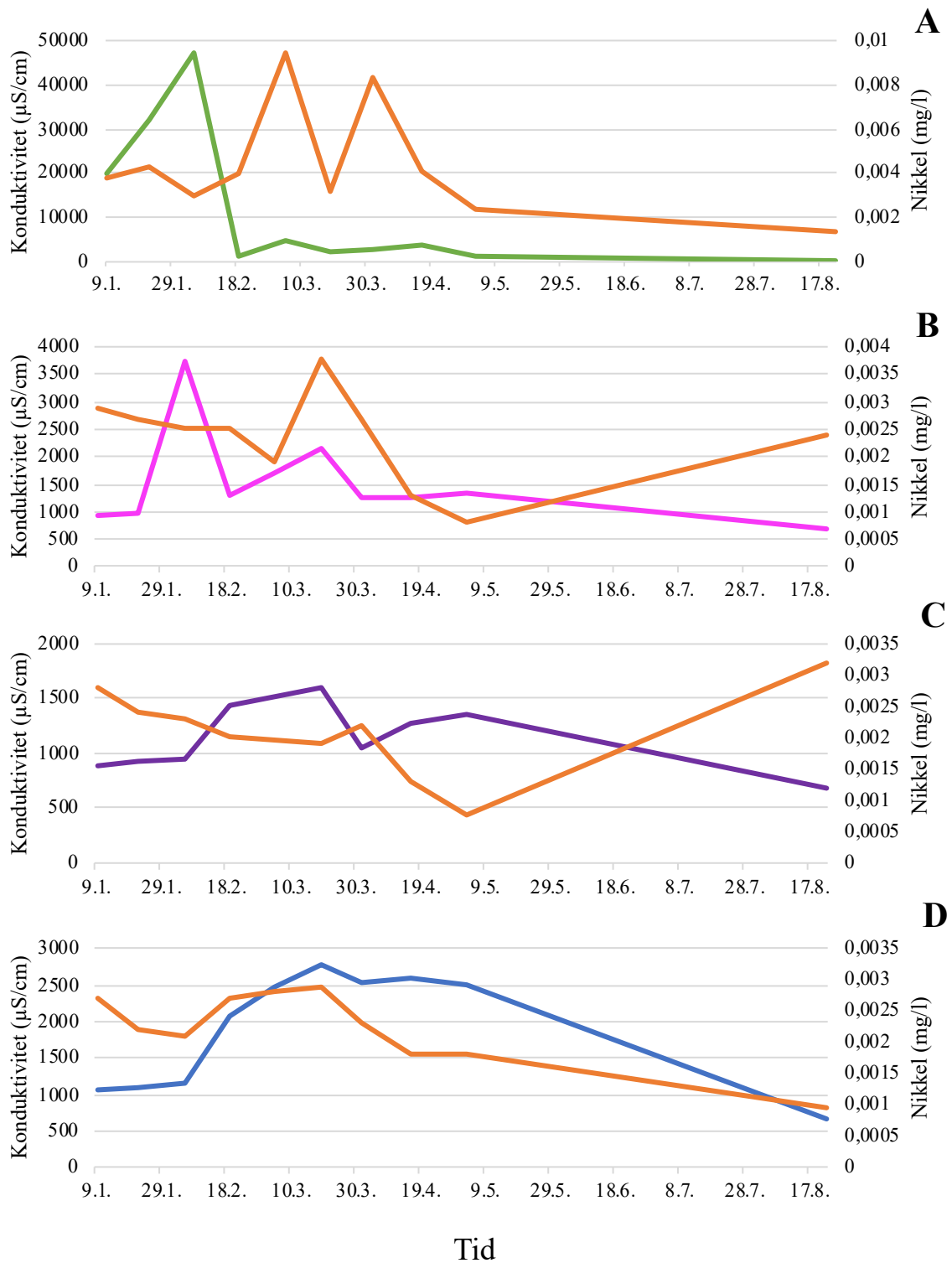
Figur 17: Nikkel og konduktivitet vist i tidsperioden 09.01.2019 til 17.08.2019 i innløpskummen (A), innløpet til rensedammen (B), Utløpet til rensedammen (C) og utløpskummen (D) til Fossbekken rensedam. Tid er vist på x-aksen, konduktivitet i µS/cm og y-aksen og nikkel i mg/l på sekundær-aksen.
