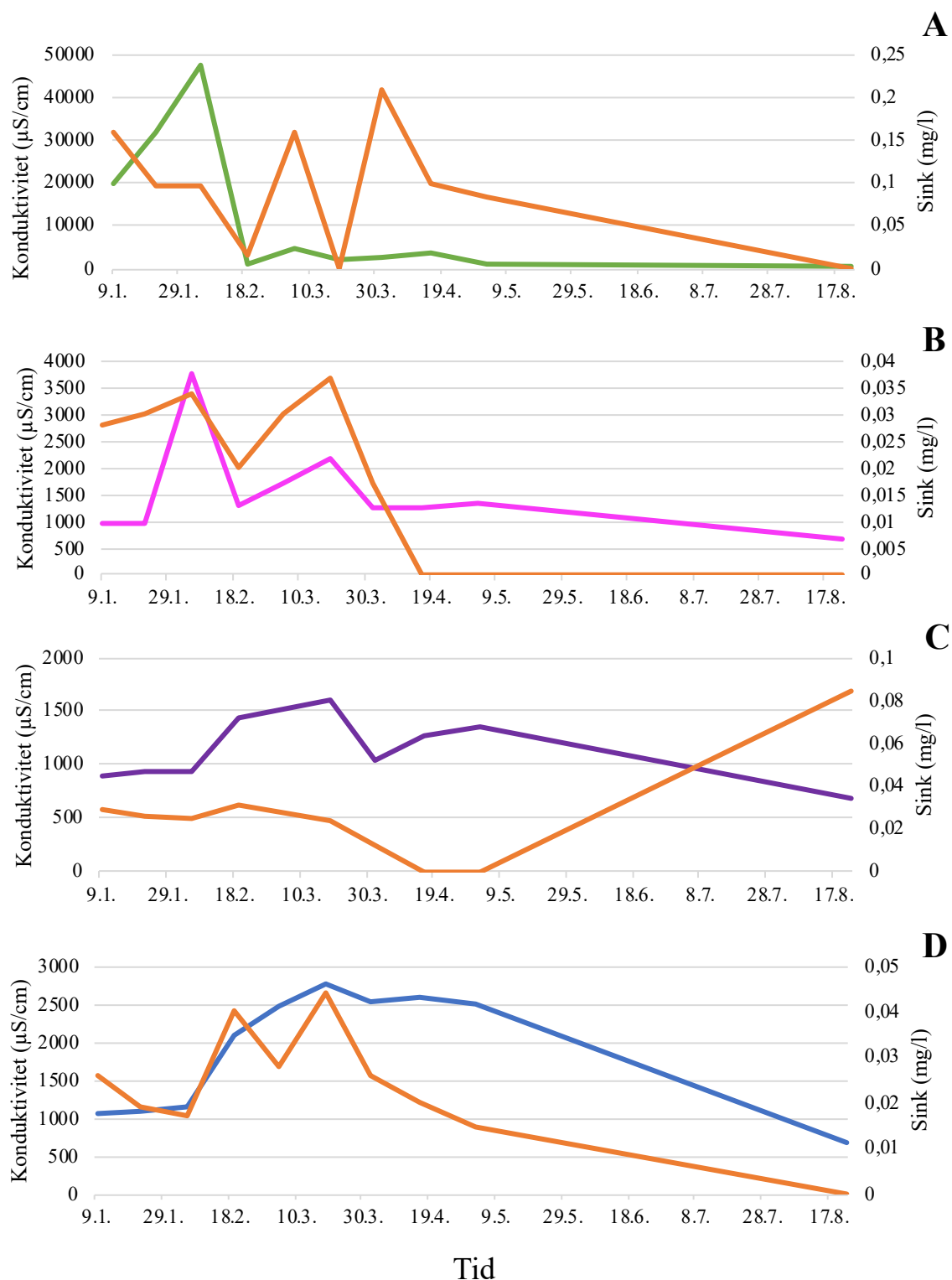
Figur 18: Sink og konduktivitet vist i tidsperioden 09.01.2019 til 17.08.2019 i innløpskummen (A), innløpet til rensedammen (B), Utløpet til rensedammen (C) og utløpskummen (D) til Fossbekken rensedam. Tid er vist på x-aksen, konduktivitet i µS/cm og y-aksen og sink i mg/l på sekundær-aksen.
