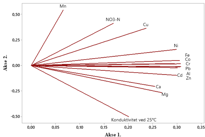
Figur 16: PCA- analyse. Loading plot A representerer innløpskummen til Fossbekken rensedam. loading plot B representerer innløpet til rensedammen, loading plot C representerer utløpet til rensedammen og loading plot D representerer utløpskummen.
