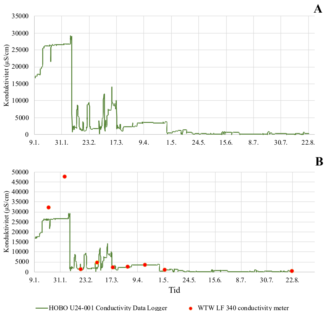
Figur 12: Konduktivitet (temperaturjustert) for innløpskummen til Fossbekken rensedam, i analyseperioden 9. januar 2019 til 22. august 2019. Konduktivitet ble registrert hver time gjennom hele døgnet i prøveperioden, vist i figur A. Figur B viser i tillegg til logget data også manuelle feltmålinger med WTW LF 340 konduktivimeter. Feltemålingene er lagt inn for å sammenligne og validere konduktivitet gjennom prøveperioden. Analyseperioden er angitt på x-aksen og konduktivitet i µS/cm er angitt på y-aksen.
