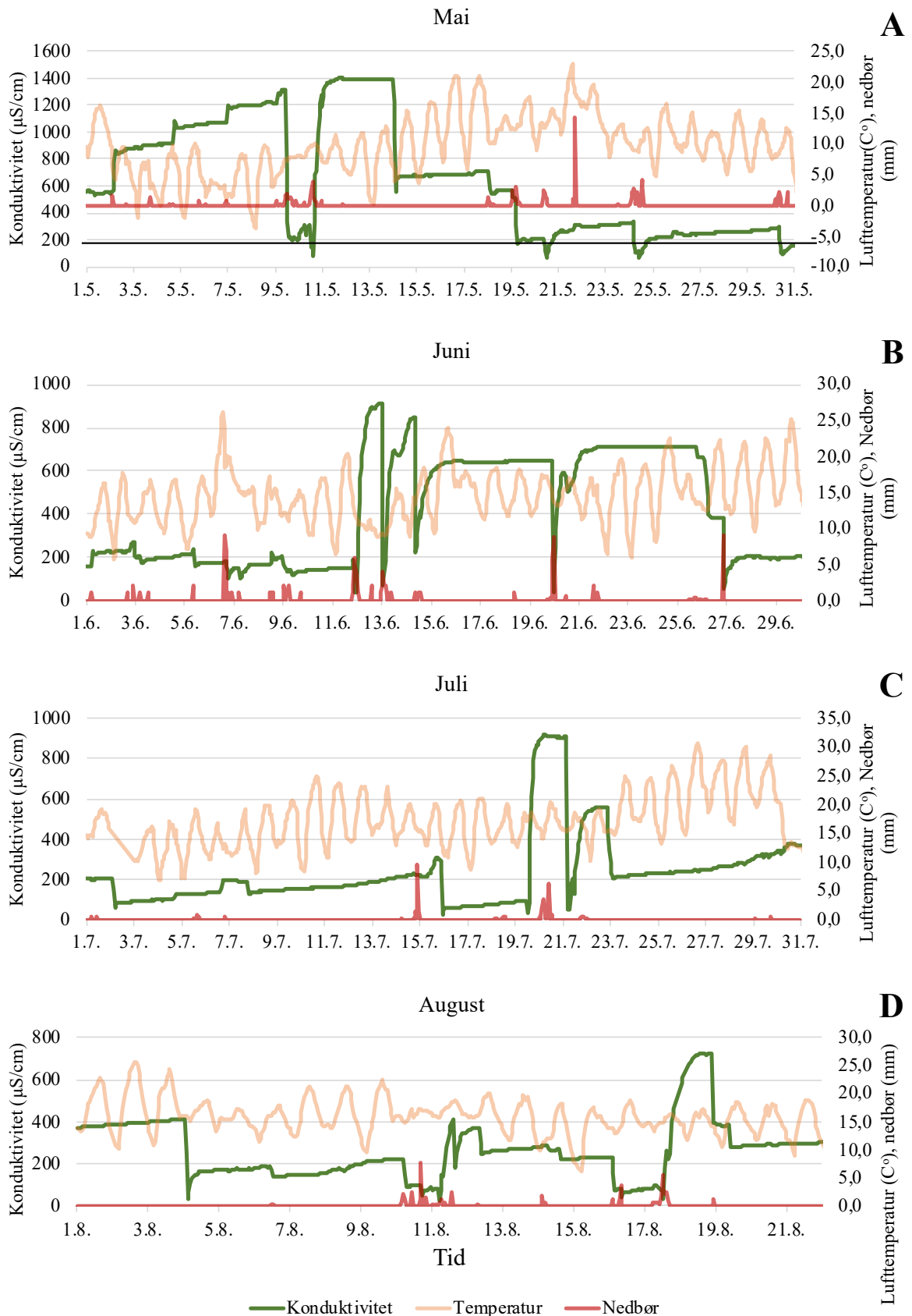
Figur 1: Månedlig fremvisning av konduktivitet og metrologiske data fra Fossbekken rensedam i tidsperioden januar 2019 til august 2019. Konduktivitet og metrologiske data ble registrert hver time gjennom hele analyseperioden. Metrologiske data lufttemperatur og nedbør er fremvist med konduktivitet i individuelle figurer for hver måned. Metrologiske data er hentet fra BIOKLIM værstasjon Ås (universitet, 2020). Tid er angitt på x-aksen, konduktivitet i \mu\text{S}/\text{cm} på y-aksen og metrologiske data på sekundær-aksen.
