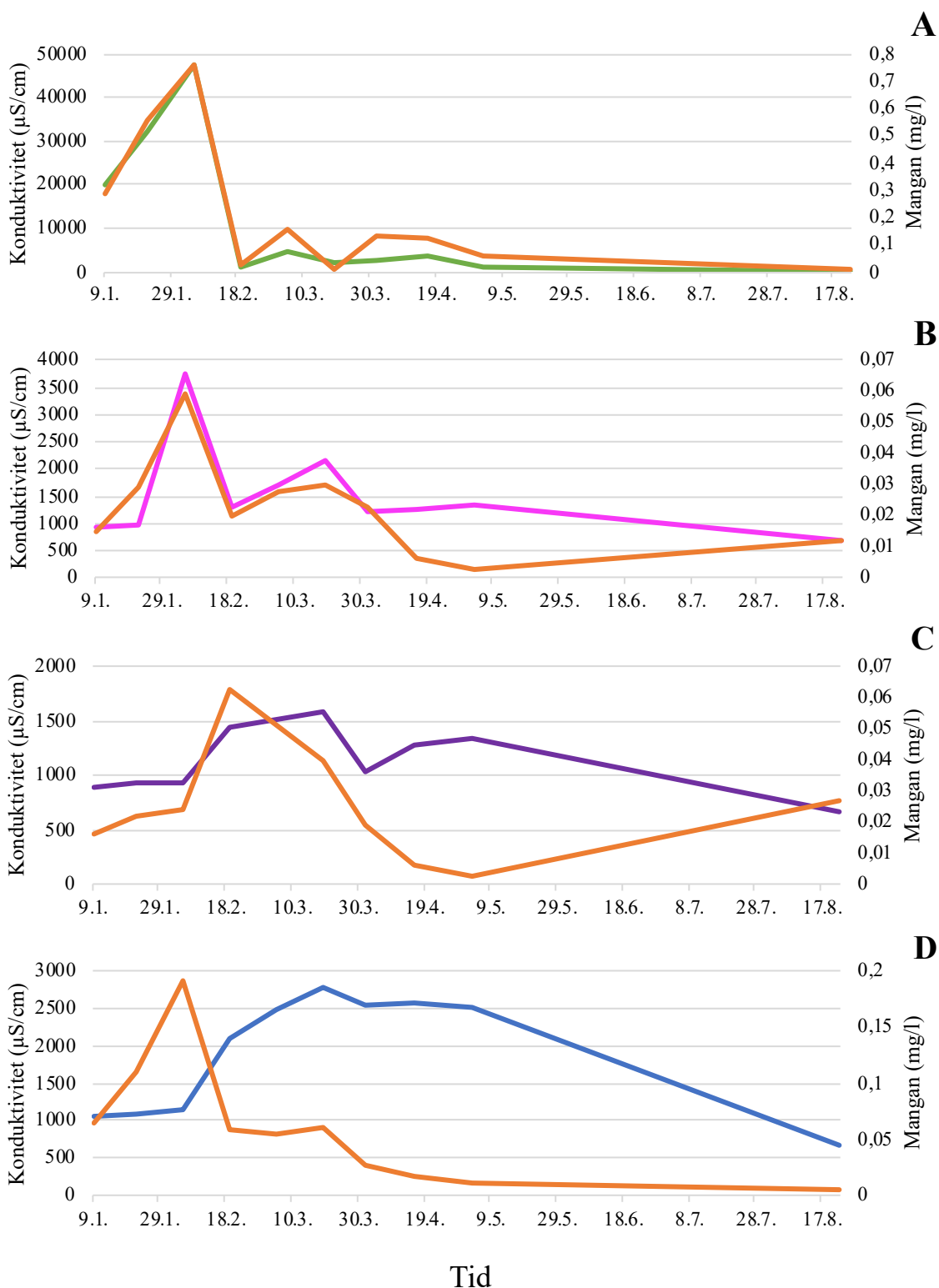
Figur 12: Mangan og konduktivitet vist i tidsperioden 09.01.2019 til 17.08.2019 i innløpskummen (A), innløpet til rensedammen (B), Utløpet til rensedammen (C) og utløpskummen (D) til Fossbekken rensedam. Tid er vist på x-aksen, konduktivitet i \mu\text{S/cm} og y-aksen og mangan i \text{mg/l} på sekundær-aksen.
