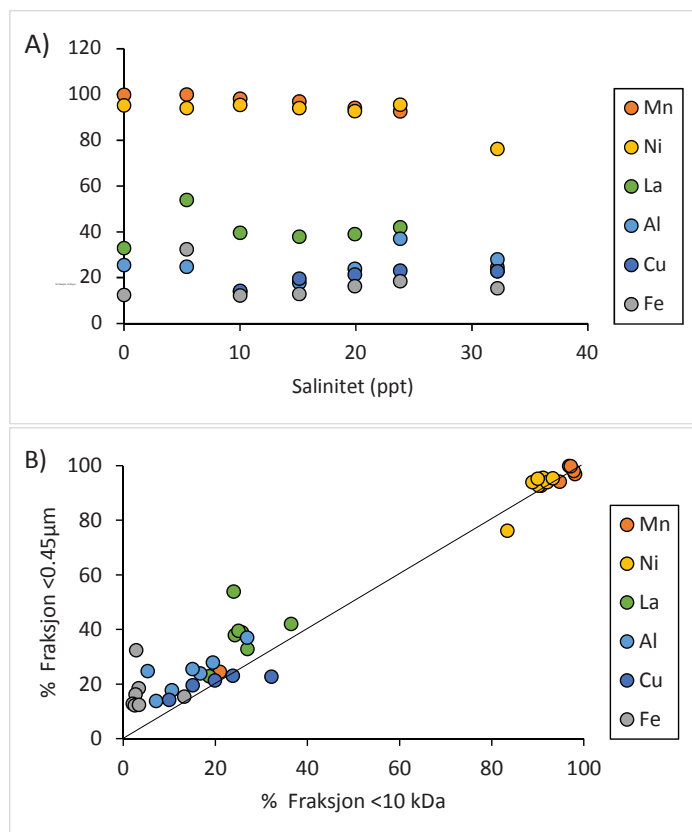
Figur 20 A) Andel spormetaller i løst fraksjon (%) i vann med ulik saltholdighet og B) sammenhengen mellom % fraksjon <10kDa og % fraksjon <0.45μm i vann etter innblanding av sjøvann i vann fra Stordalsbekken.
