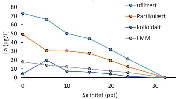
Figur 19 Fordeling av ulike tilstandsformer av A) Fe, B) Ni, C) Cu og d) La i vann ut fra rensanlegget tilsatt sjøvann til ulik saltholdighet.
