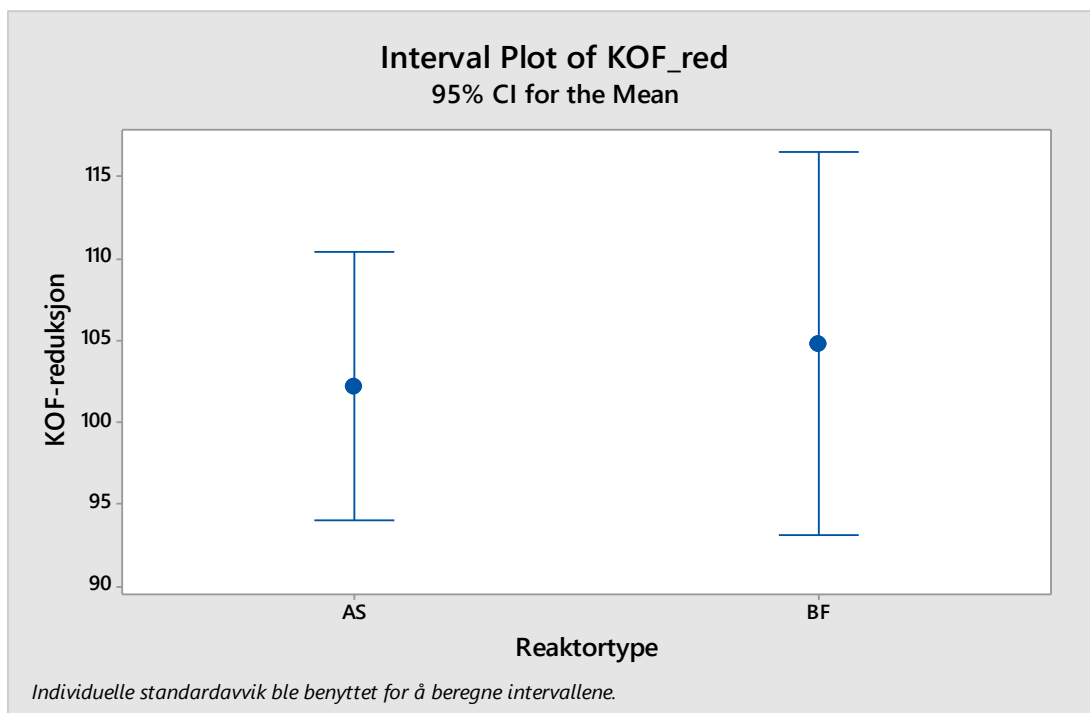
Figur 53: Intervallplot for KOF-reduksjon i aktivslam- og MBBR-reaktorene gjennom oppstartsperioden på fire uker. Den blå prikken markerer gjennomsnittet av alle verdiene fra hver reaktortype (AS er aktivslam og BF er MBBR). Øvre og nedre strek markerer et 95% konfidensintervall.
